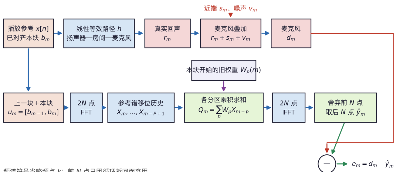
图39 PBFDAF：参考历史、有效输出与受控权重更新
