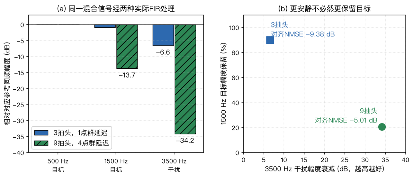
图 47: E11-19 中实际 FIR 处理后的 PCM 结果。500 Hz 与 1500 Hz 组成目标，3500 Hz 为噪声；两滤波器的 500 Hz 解析增益均为 1，四个 WAV 使用共同增益 0.8。(a) 展示三个频率的同频幅度比，目标以干净 PCM 为参考，干扰以混合输入 PCM 为参考。(b) 比较 3500 Hz 干扰抑制与 1500 Hz 目标保留，标注对齐后的总 NMSE；两滤波器延迟分别为 1 点和 4 点。频率测量与表中 PCM 口径一致；它显示数学合成三音模型中的取舍，不代表语音识别或主观质量排名。
