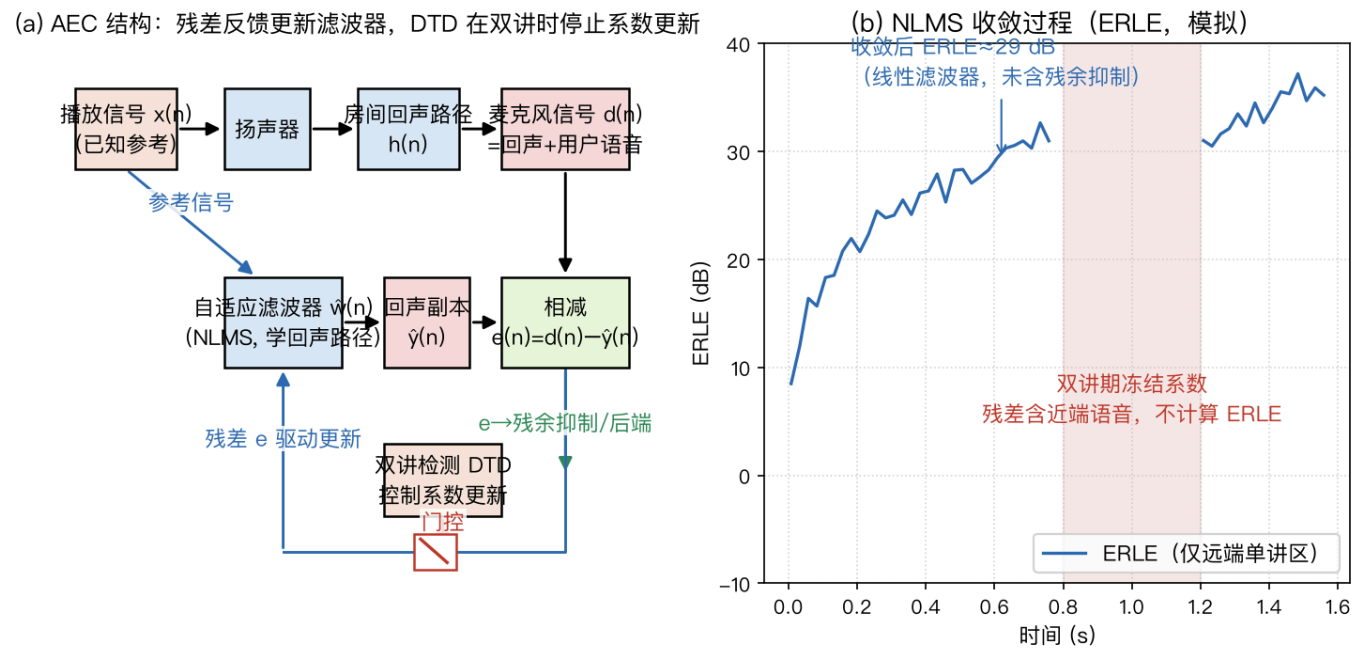
图18 (a) 给出整体结构； (b) 给出 NLMS 在模拟回声路径上的收敛曲线。仿真取 \mu = 0.5 ，回归向量按 \vec{x}(n) = [x(n), x(n - 1), \dots, x(n - L + 1)]^\top 排列，与生成回声的卷积索引一致，不额外引入一拍延迟。图中标注的是固定随机种子下 0.45 < t < 0.8 \text{ s} 远端单讲窗口的 ERLE 均值；粉色区域表示双讲期间冻结更新，该区间不统计 ERLE。
