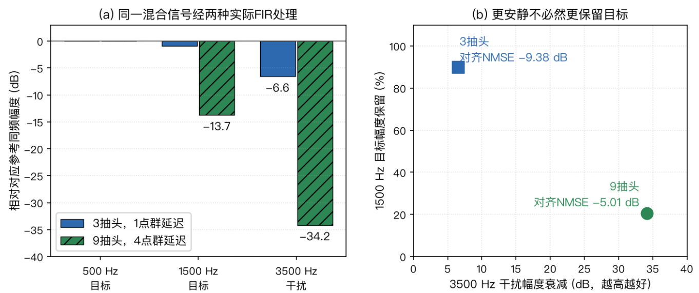
图 47: 合成三音经 3/9 抽头 FIR 的 PCM 读回；四份 WAV 共用增益 0.8，分别保留 1、4 点延迟，NMSE 评分时对齐。(a) 同频幅度比：500/1500 Hz 目标除以干净 PCM，3500 Hz 干扰除以混合 PCM。(b) 3500 Hz 抑制、1500 Hz 保留及对齐 NMSE。仅示合成取舍，不代表自然语音、ASR 或听感。
