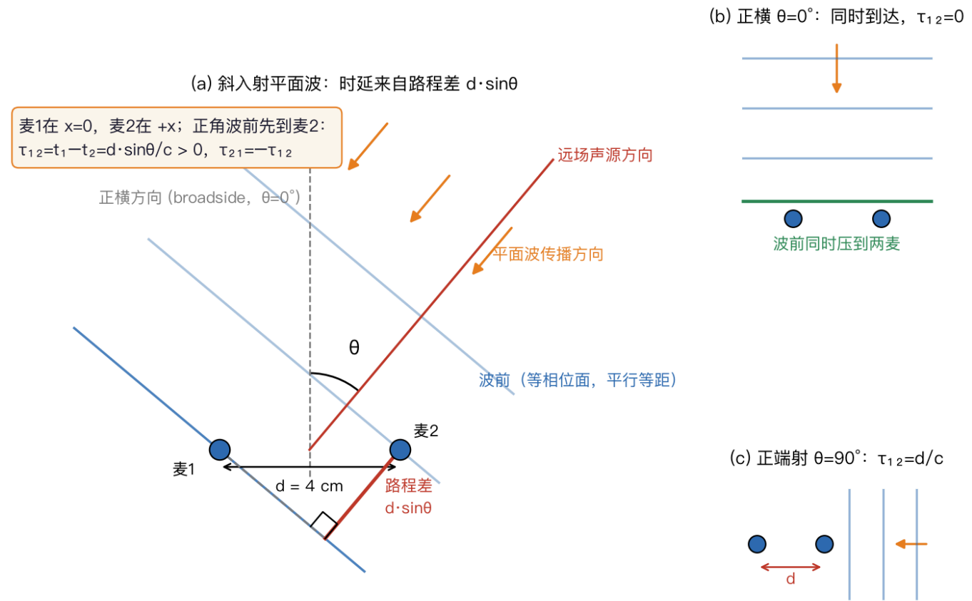
图2 时延的几何来源与角度约定（示意）
