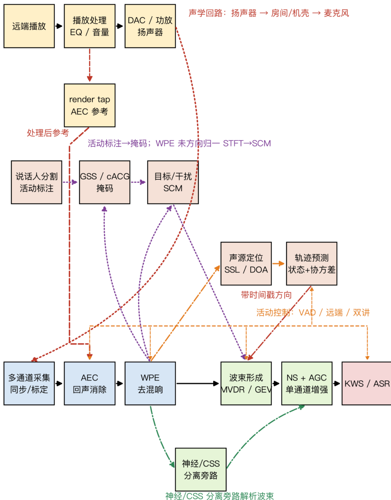
图 23 按较完整的语音交互系统绘制。远端音频先经过混音、均衡和音量控制；AEC 的 render tap 取在这些播放处理之后、DAC/功放之前，扬声器经房间和机壳耦合回麦克风形成声学回路。虚线表示活动控制，实线表示音频、特征或统计量依赖。图中 AEC 的“最
