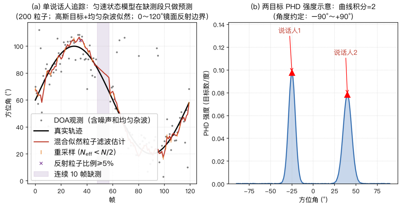
图22 (a) 中，灰点为逐帧 DOA 观测，黑线为正弦真值轨迹，红线为粒子滤波估计，紫色阴影标出连续 10 帧缺测，橙色竖线表示有效粒子数低于 N/2 后执行了系统重采样；紫色叉号只标出该帧预测后至少 5% 粒子越界并被镜面反射的时刻，避免用“任一粒子越界”放大单个尾部样本。缺测段没有似然更新，轨迹只由匀速状态模型与过程噪声外推； 0^\circ 与 120^\circ 是采用反射规则的有限扇区边界。(b) 在 -25^\circ 和 +40^\circ 附近设置两个强度峰，用于说明多目标强度函数。峰数只能近似用于提取人数，严格定义见 § 9.3。
