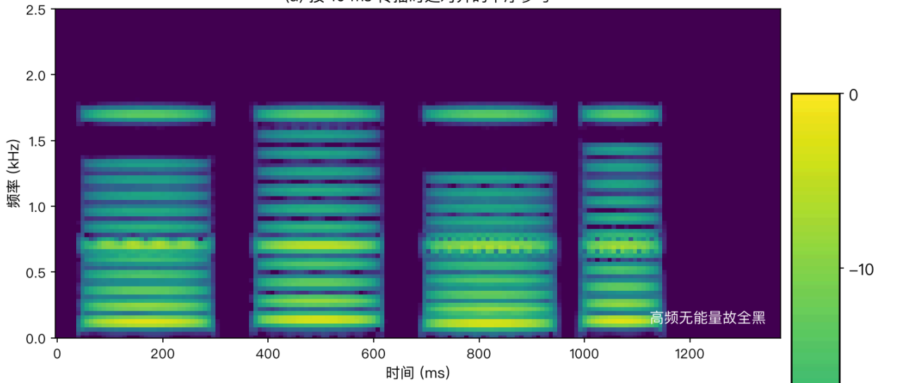
图21 WPE 去混响效果（本书单通道仿真）
