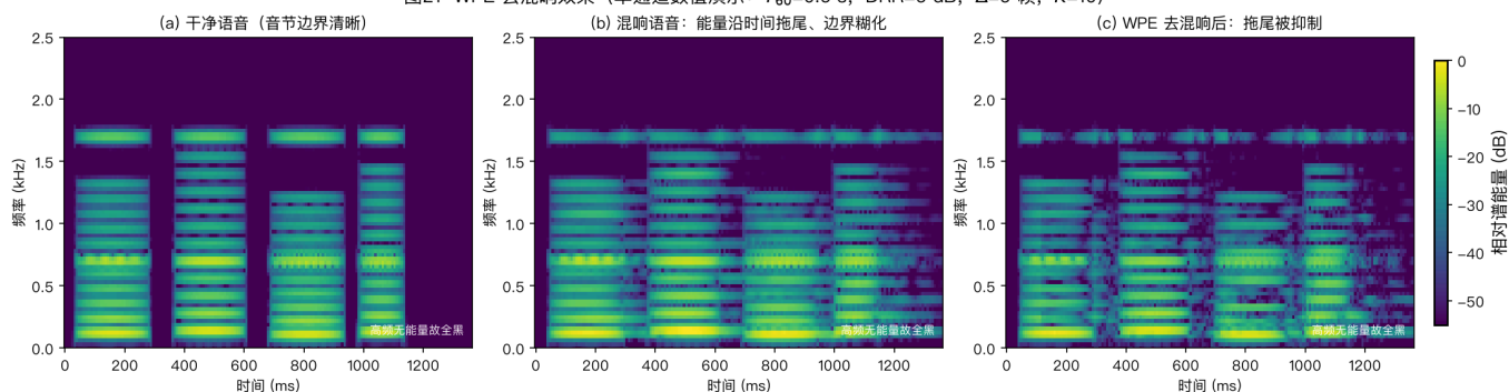
图21 WPE 去混响效果（单通道数值演示： T_{60}=0.6 s, DRR=6 dB, \Delta=6 帧, K=10 ）
