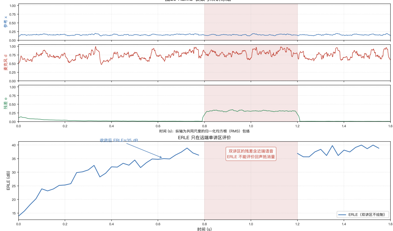
图29 NLMS 收敛与双讲冻结
