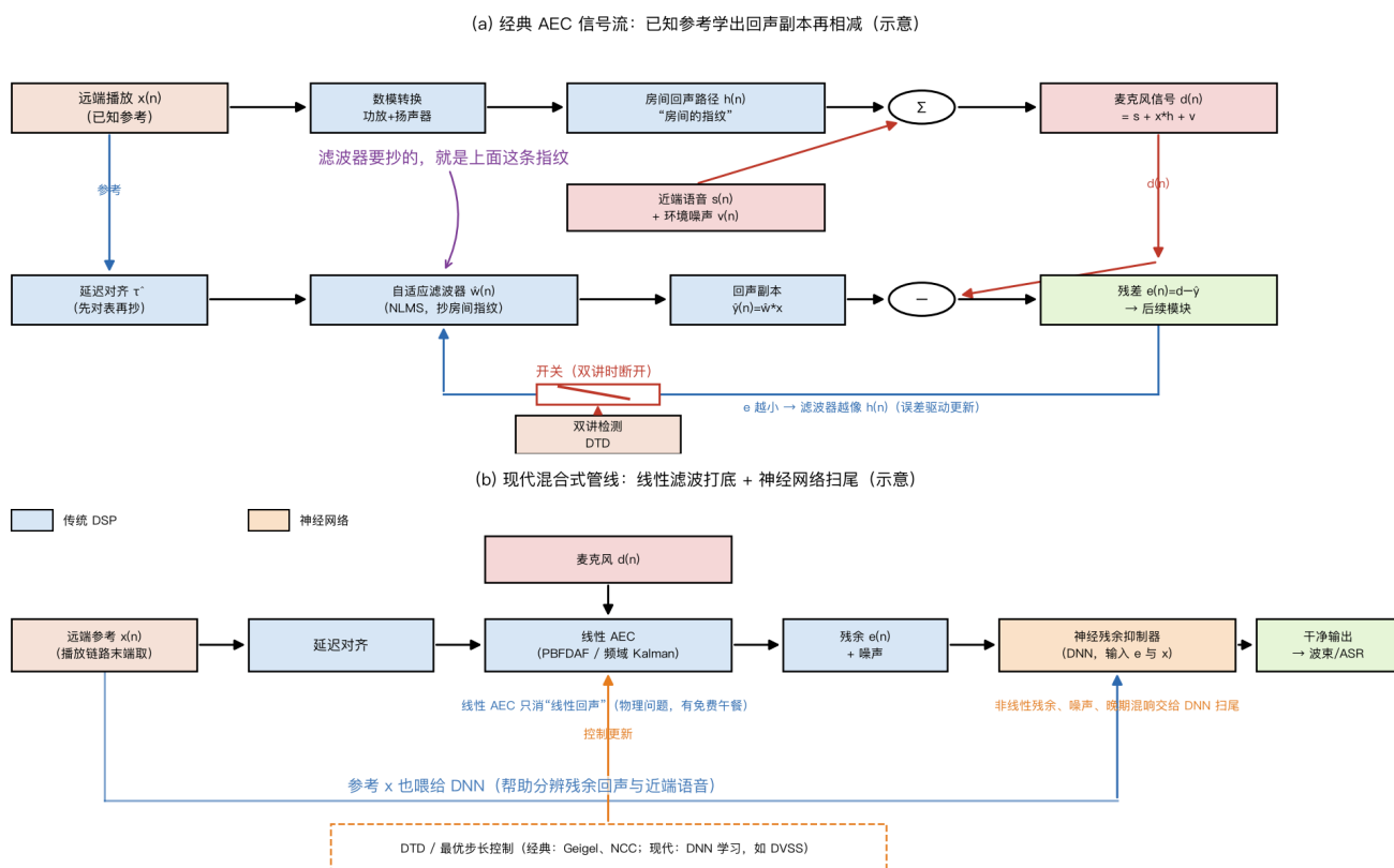
图20 AEC 系统管线：从经典自适应结构到现代混合式（示意）
