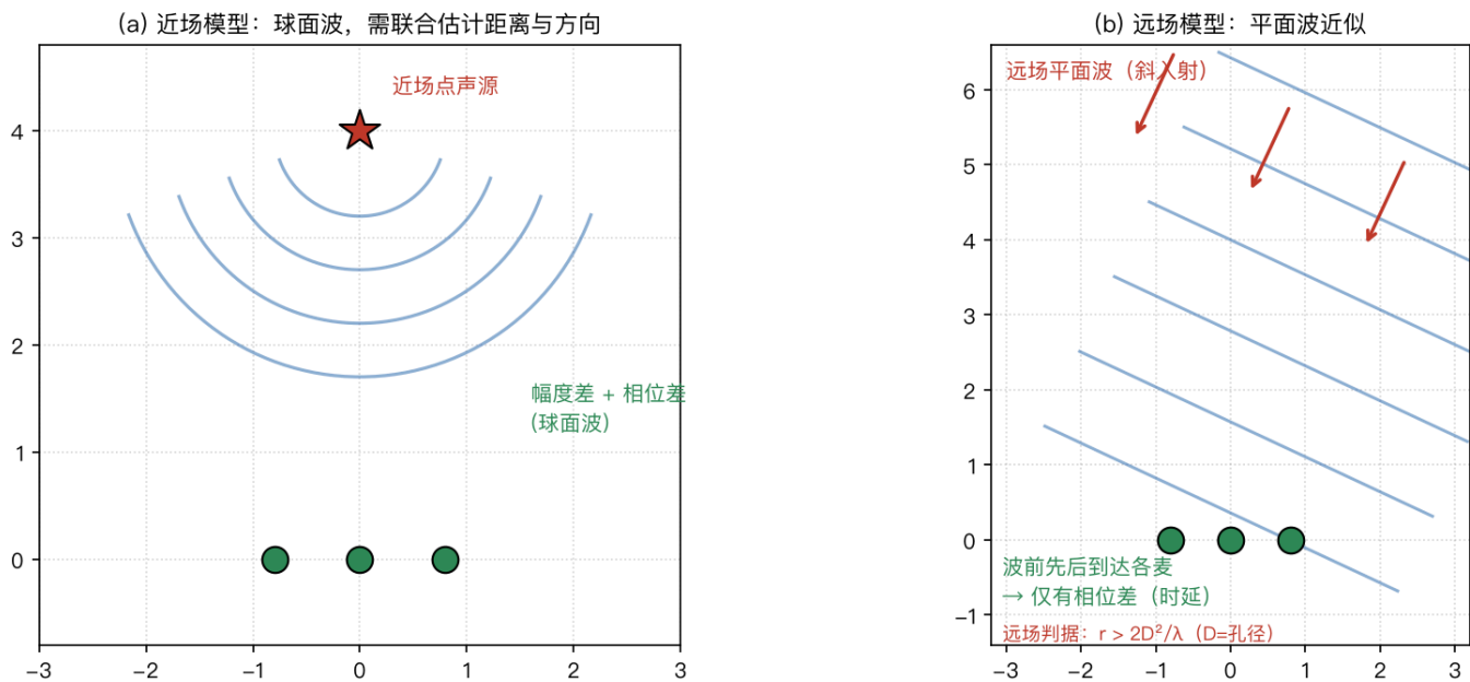
图 3 对比两种波前：近场采用球面波模型，各通道同时存在传播时延和幅度差；远场近似为平面波，传播模型主要由方向决定。这是下一节远场向量模型的前提。
