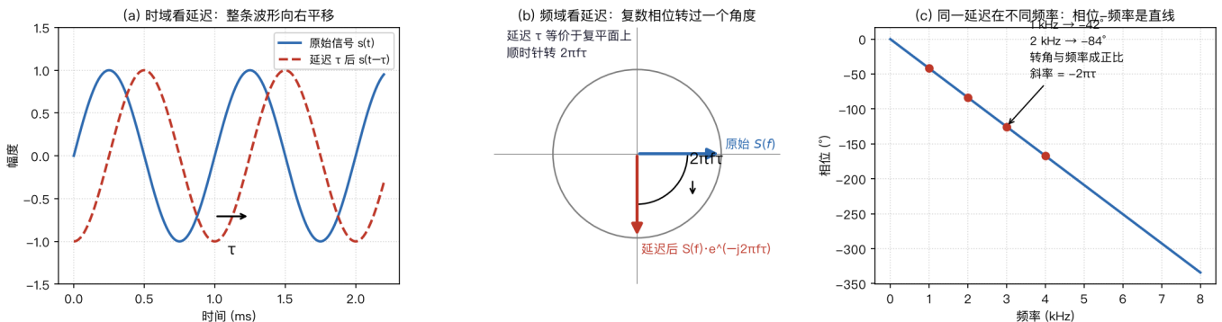
图4 时延为什么变成 e^{-j2\pi f \tau} ：几何直觉（4 cm 麦距、正侧向、 \tau=0.116 ms）
