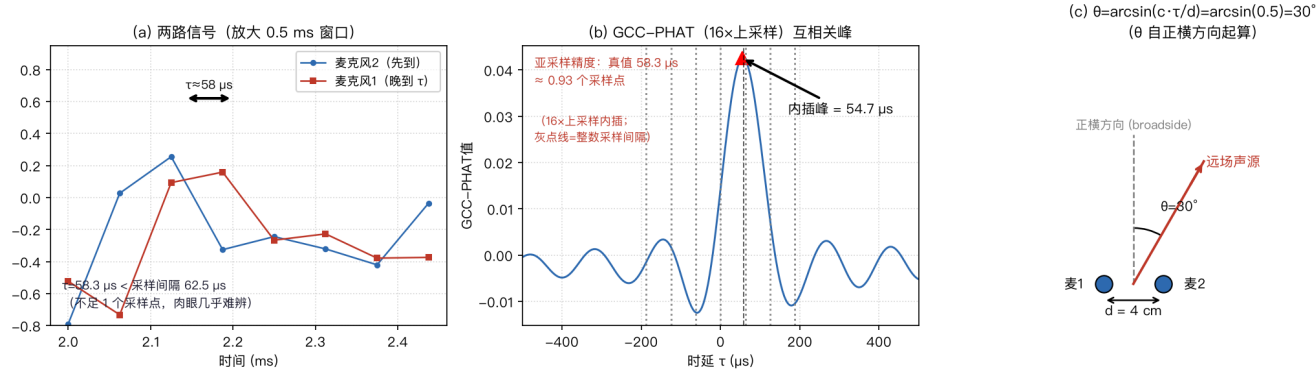
图12 GCC-PHAT 声源定位原理：亚采样时延估计（模拟）
