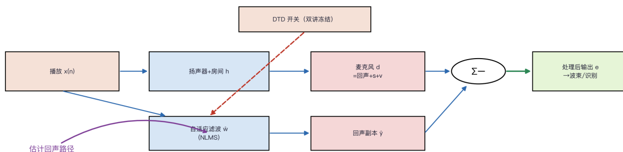
图27 AEC 结构：根据播放参考估计回声，再从麦克风信号中相减
