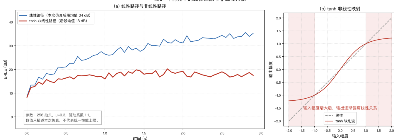
图31 本仿真中的线性匹配与非线性失配
