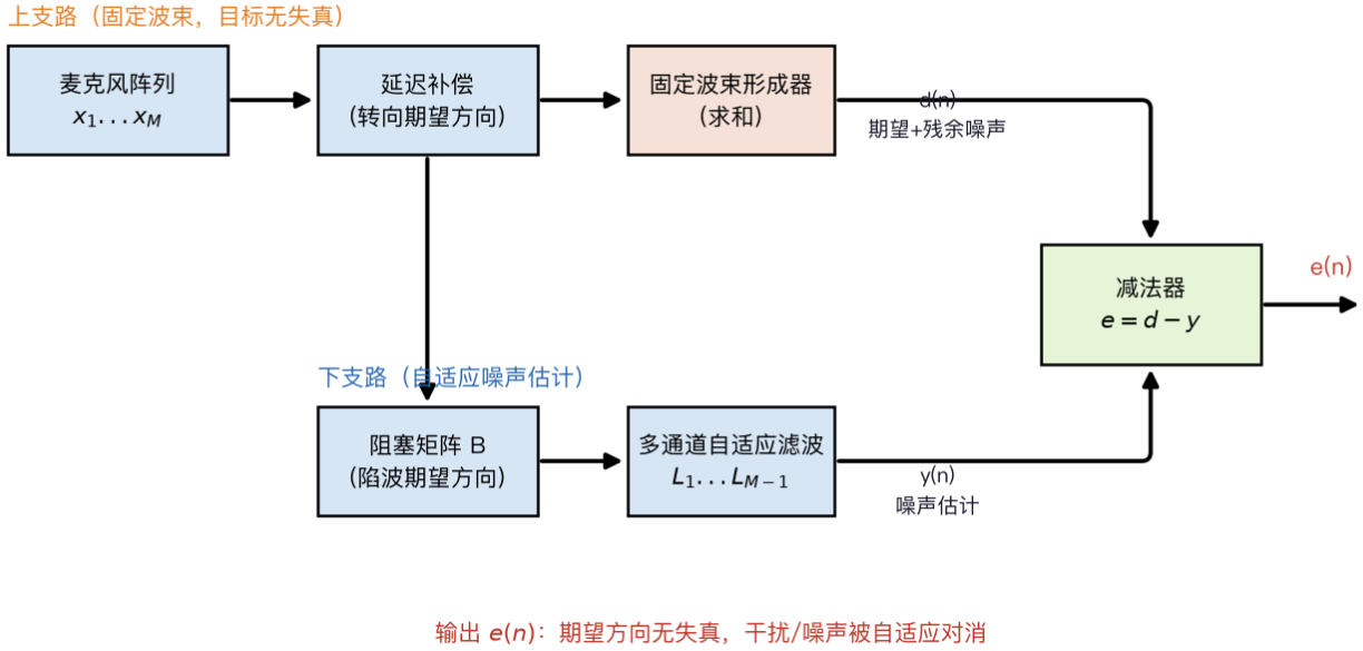
图17 GSC（广义旁瓣对消器）结构框图
