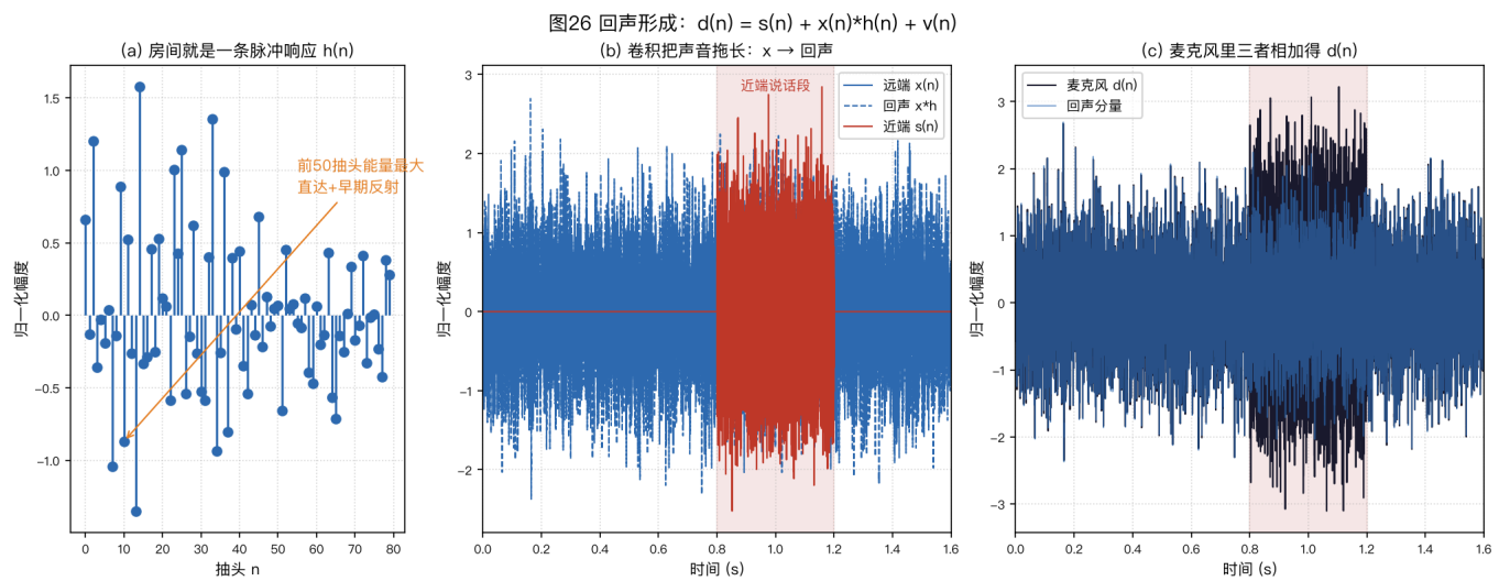
图26 (a) 用冲激响应 h(n) 表示房间路径，前部主要包含直达声和早期反射，后部是逐渐衰减的拖尾。(b) 给出远端参考、卷积后的回声和 0.8~1.2 s 的近端语音。(c) 显示三者 in 麦克风信号 d(n) 中叠加。AEC 根据参考估计回声分量，再从 d(n) 中减去该估计。
