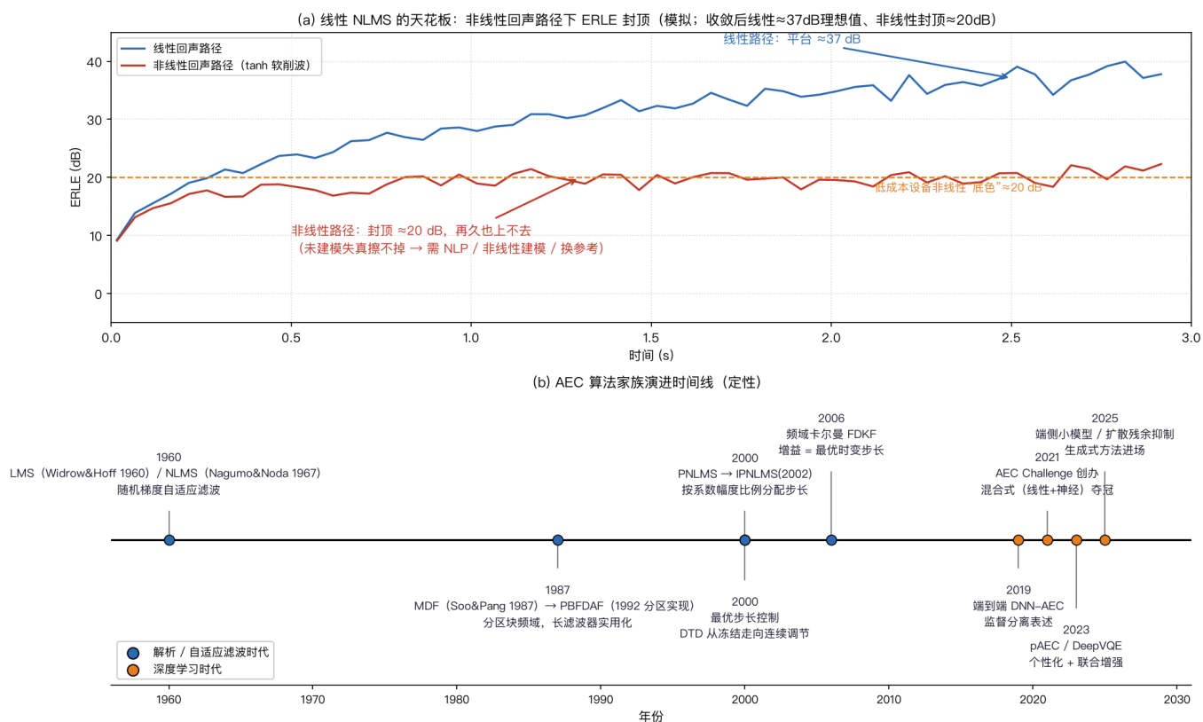
图19 (a) 比较该脚本配置下的线性路径与 tanh 非线性路径。约 37 dB 和 19~20 dB 只适用于图中的输入、路径和统计区间。(b) 列出 LMS/NLMS、FDKF 和 AEC Challenge 等发展节点，用于说明线性估计、自适应控制与学习型残余抑制的分工变化。
