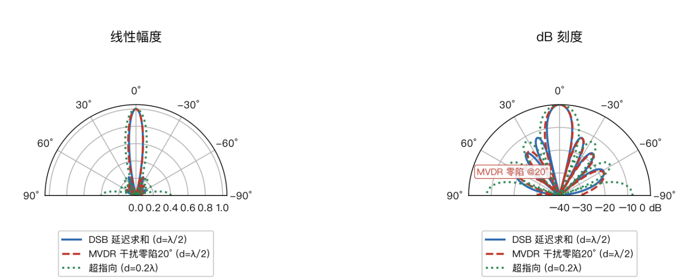
图16 8元ULA 0°指向波束图对比：DSB / MVDR(零陷@20°) / 超指向 (f=2kHz, d=λ/2, c=343m/s, 上=0°正横, 模拟)
