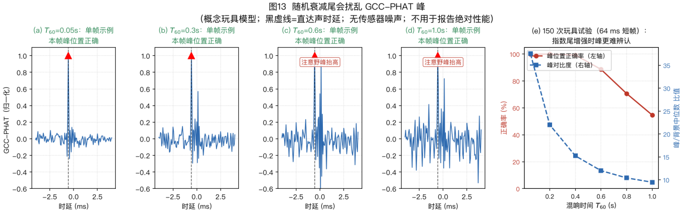
图示说明： 图13(a)–(d)是随机衰减尾模型的单帧样例，旁峰位置受随机实现影响；图13(e)汇总 150 次玩具试验。该图用于说明衰减尾增强时主峰对比度和选峰正确率下降，不代表镜像法房间仿真或实测性能。
