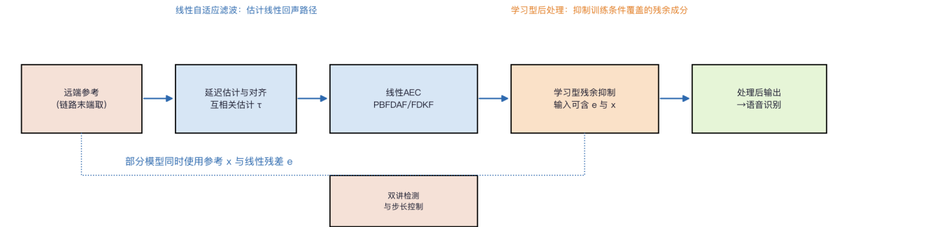
图32 线性回声消除与残余抑制：按系统条件选择模块 (a) 一种常见的混合处理流程
