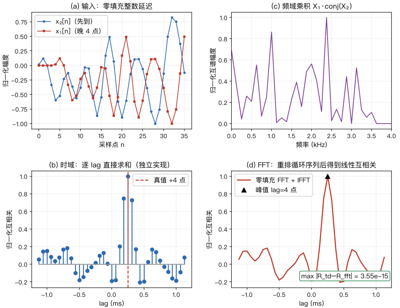
图 33 (a) 给出零填充整数延迟信号; (b) 按定义逐个时延直接求和; (c) 计算频域乘积 X_1 X_2^* ; (d) 用零填充 FFT 和 IFFT 得到线性互相关。时域与频域由独立代码计算, 图中给出最大数值误差。该图对应 \Phi(f) = 1 的普通互相关, 不包含 PHAT 加权。
