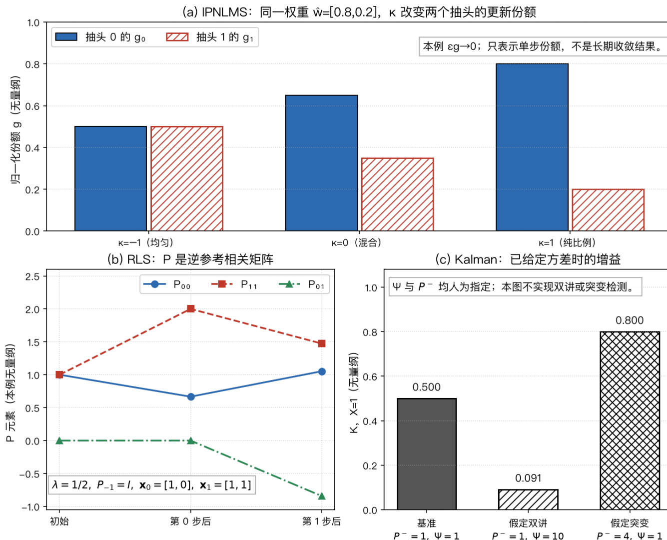
图38 IPNLMS、RLS 与 Kalman：三种不同的更新状态
