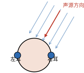
图1 人类双耳定位线索：几何 ITD 与双重理论的适用边界
