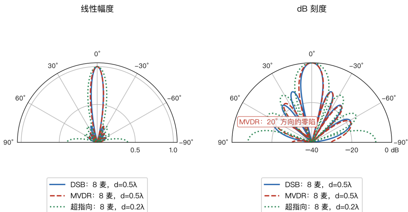
图16 8 麦线阵的三种波束：两种阵距，不能作为同条件性能排名 DSB/MVDR: d = 0.5\lambda ; 超指向: d = 0.2\lambda ; 目标方向 0^\circ 、响应均为 1; MVDR 干扰 20^\circ
