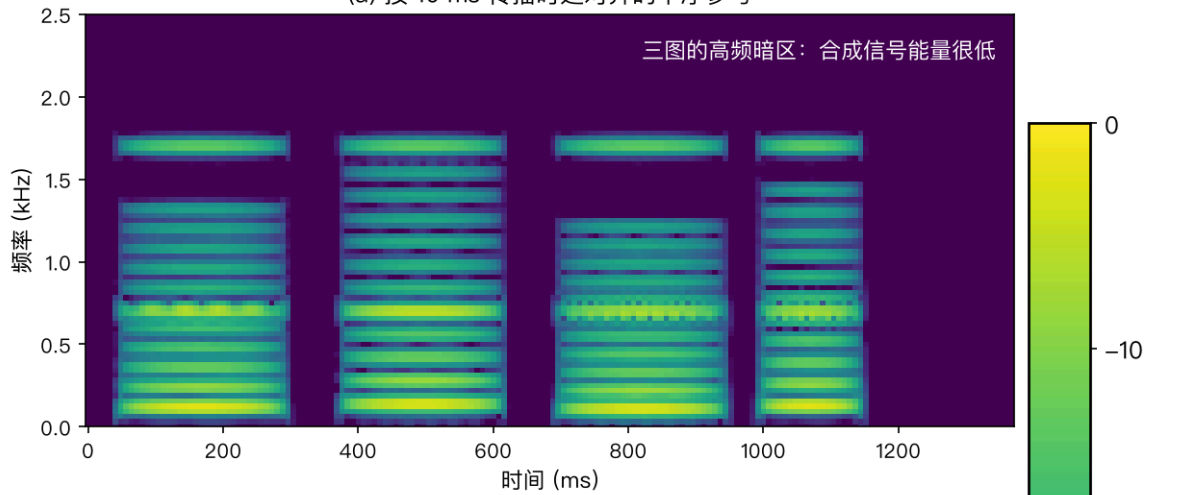
图21 WPE 去混响效果（本书单通道仿真）
