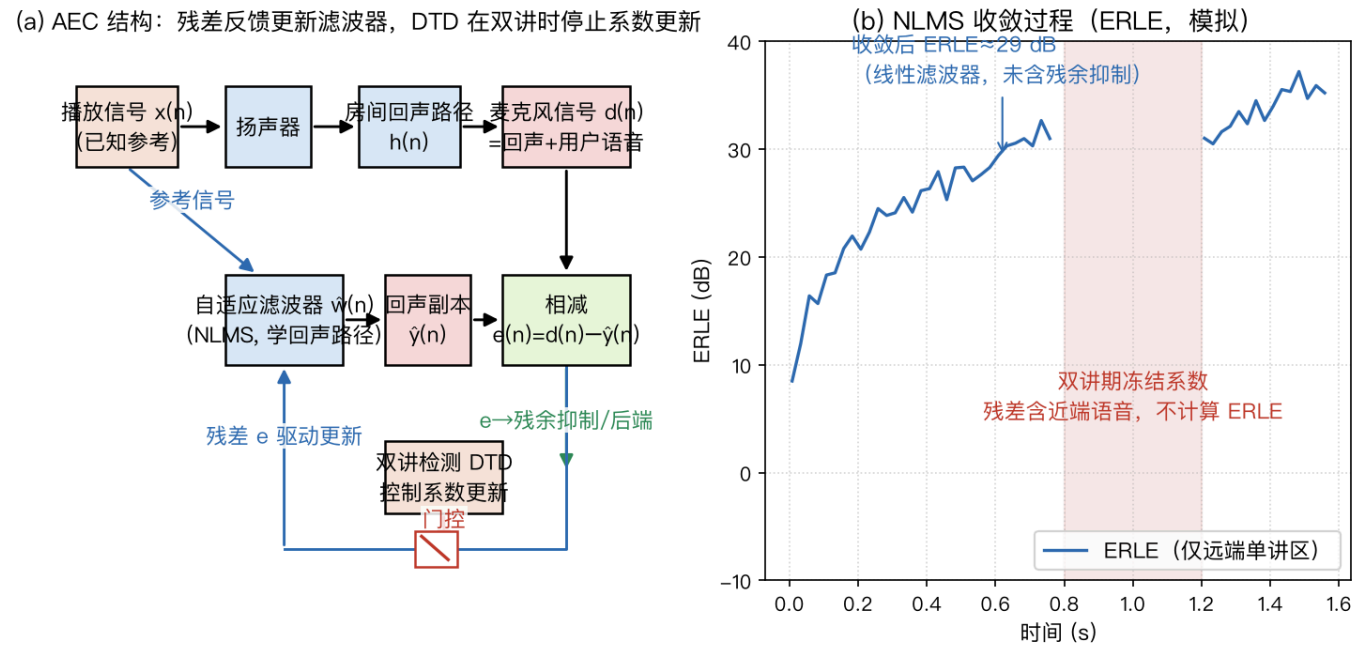
图18 声学回声消除 (AEC) 原理
