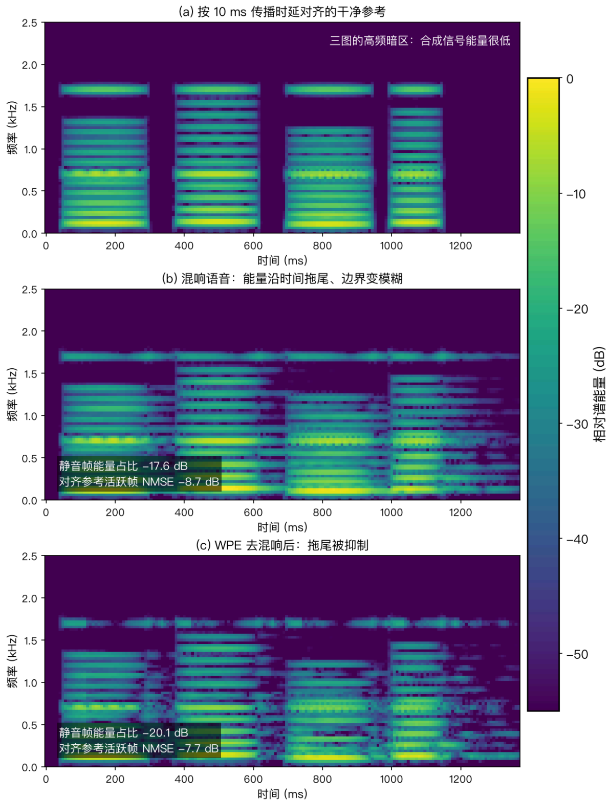
图21 WPE 去混响效果（本书单通道仿真）
