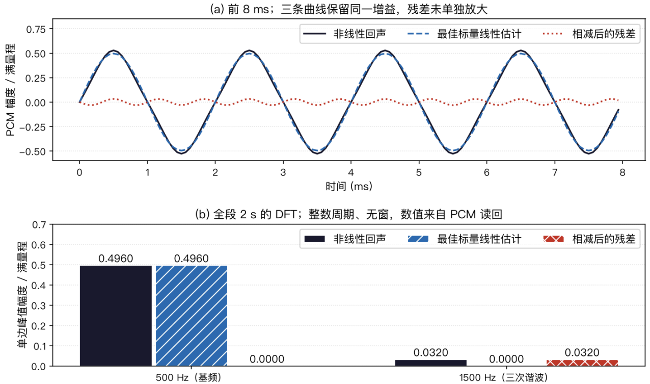
图36 三次非线性留下线性估计无法表示的谐波（合成反例）
