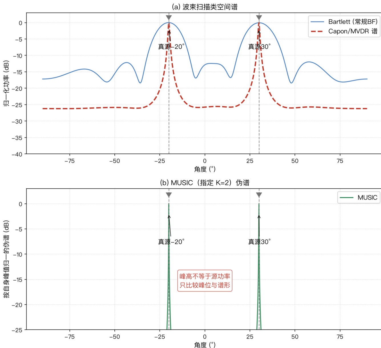
图11 两信号源( -20^\circ , 30^\circ ) DOA空间谱估计对比 (8元ULA, 每阵元设定总输入SNR=20dB, 400快拍, 模拟)
