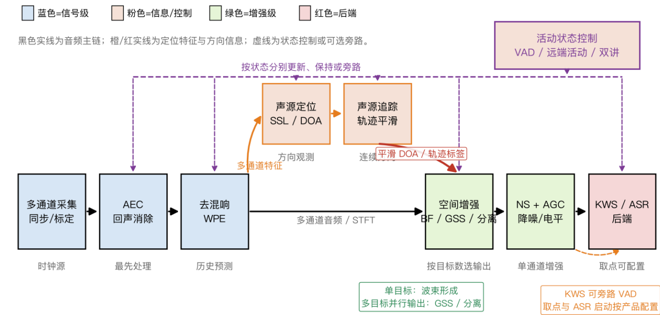
图23 远场语音前端：音频主链、方向反馈、状态控制与可选旁路
