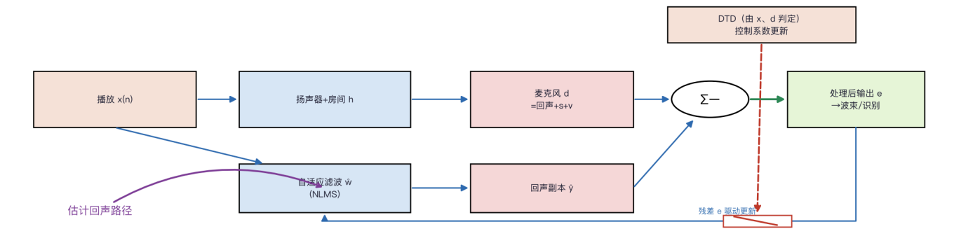
图27 AEC 结构：根据播放参考估计回声，再从麦克风信号中相减
