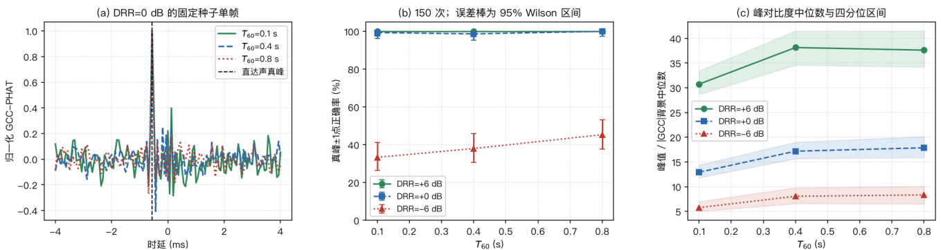
图13 GCC-PHAT 的两因素实验：随机尾时长 T_{60} 与尾能量 DRR 直达能量=1；两通道独立随机尾按目标 DRR 固定总能量；64 ms 帧；无加性噪声；本书仿真
