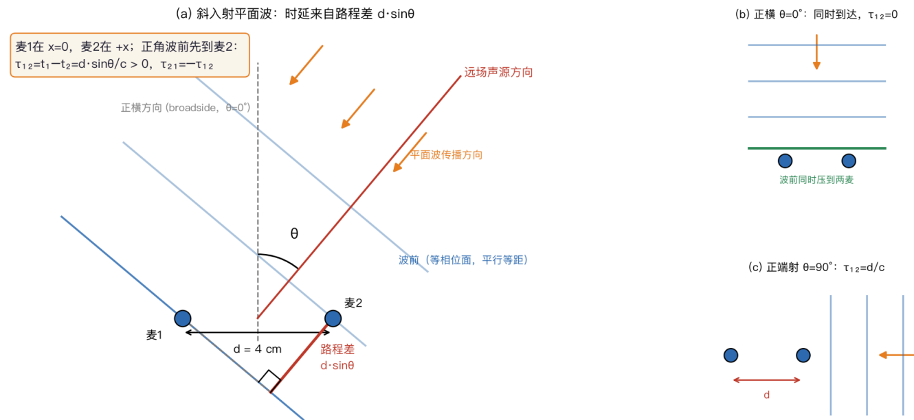
图2 时延的几何来源与角度约定（示意）
