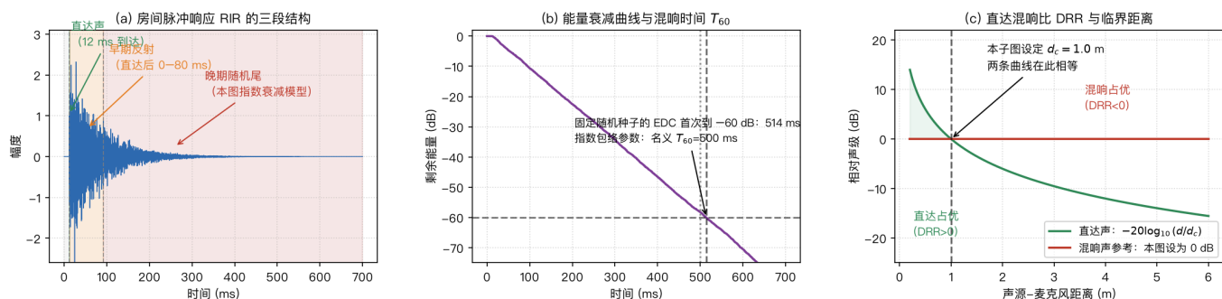
图5 房间脉冲响应、能量衰减与直达混响比（本书仿真）
