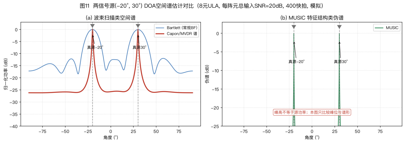
图 11 在同一个两源仿真 (−20°、30°) 中比较 Bartlett、Capon 和 MUSIC。条件为 8 元半波长 ULA、每阵元总输入 SNR 20 dB、400 个快拍, 两源相隔 50°; 这个较容易的条件只展示三种谱形, 不检验最小可分辨角度。Bartlett 与 Capon 按各自的标准空间谱公式计算; MUSIC 给出伪谱, 峰高不是功率。只有在源间隔、信噪比、快拍数、源数和阵列失配都明确时, 才能用重复试验比较分辨成功率。
