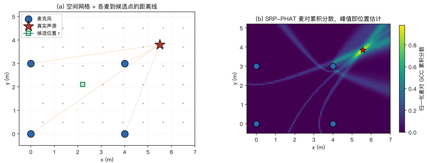
图14 SRP-PHAT 定位过程（独立米级分布式阵列例） 4 m × 3 m 四麦；源(5.5, 3.8) m；c=343 m/s；高斯峰σ=166.7 μs；90×68网格
