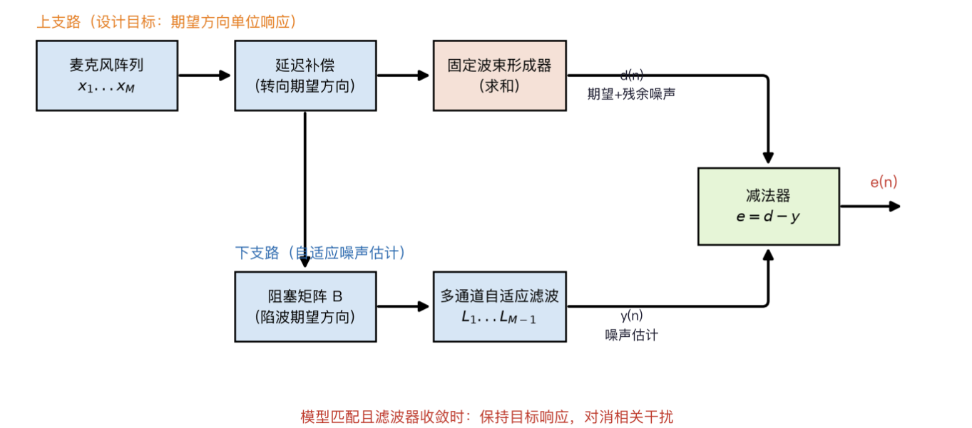
图17 GSC（广义旁瓣对消器）结构框图
