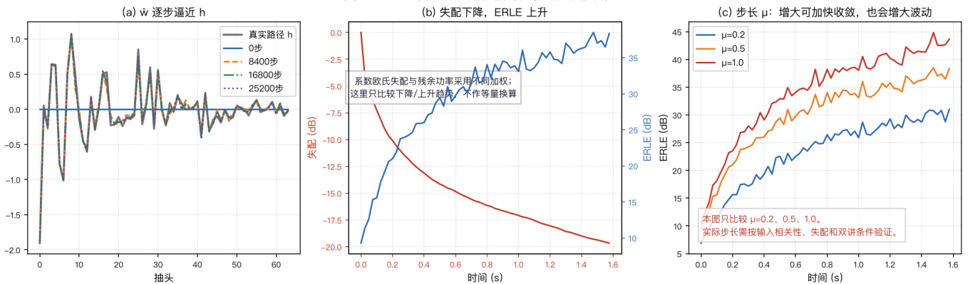
图28 NLMS 自适应：路径估计逐步逼近真实响应
