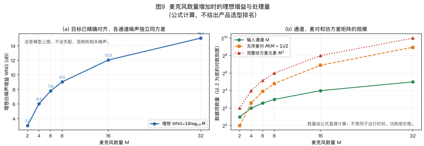
图 9 (a) 在目标精确对齐、各通道噪声独立同方差的条件下，按 10 \log_{10} M 画出理想 DSB 白噪声增益。(b) 分别按 M 、 M(M-1)/2 和 M^2 计算输入通道、无序麦对与完整协方差矩阵的元素数量。右图的纵轴采用以 2 为底的对数刻度。这些数量用于说明数据结构怎样随 M 增长，不等同于具体实现的运行时间、功耗或价格。
