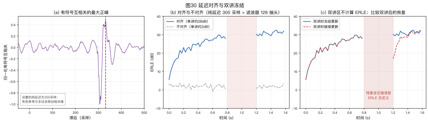
图30 (a) 在前 4000 个样本上计算参考与麦克风信号的有符号互相关，最大正相关峰位于约 331 个采样。仿真设置的纯延迟是 300 个采样；参考是有色信号，路径又含多个正负抽头，因此相关峰是输入自相关与整条路径共同作用的结果，不能解释成“300 加某个主抽头位置”。若改取互相关绝对值、使用广义互相关（Generalized Cross-Correlation, GCC）加权或改变参考频谱，峰值也可能改变。(b) 对齐后的远端单讲 ERLE 约为 28 dB，不对齐时约为 2 dB。本例的纯延迟超过 128 抽头滤波器的覆盖范围，因此差异较大。(c) 比较双讲期间冻结和继续更新；后者会使路径估计偏离，双讲结束后需要重新收敛。排查时应分别检查延迟估计方法和双讲控制。
