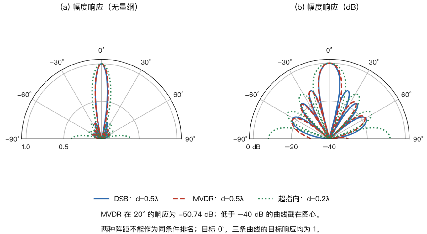
图16 8 麦线阵的固定与自适应方向图
