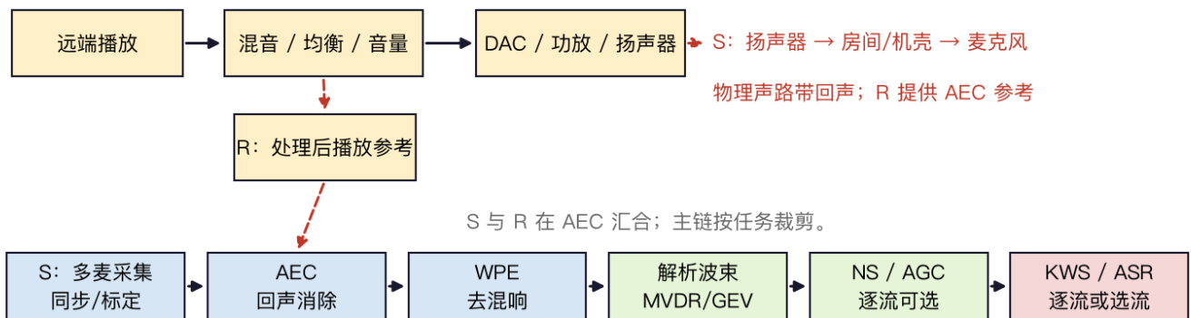
图23 播放参考、音频主链与条件支路
