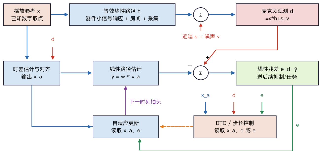
同名端口连接同一信号； \hat{w} 表示对齐后路径， h 表示从原参考到麦克风的总路径。 (b) 一类混合流程：线性估计 + 学习型残余抑制
