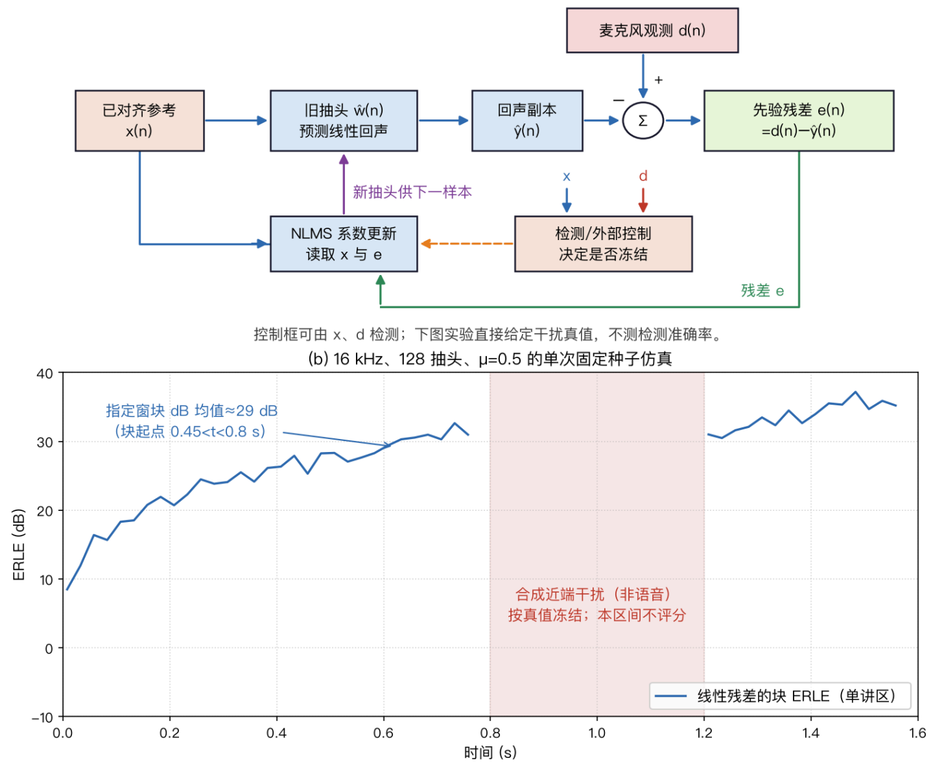
图18 (a) 从已经对齐的参考和麦克风观测开始，按旧权重预测、形成先验残差、更新权重的顺序画出控制依赖；它不是物理播放回路。
