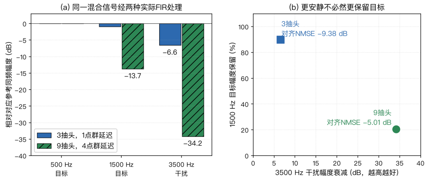
图 47: 合成三音经 3/9 抽头 FIR 的 PCM 读回；四份 WAV 共用增益 0.8，分别保留 1、4 点延迟，NMSE 评分时对齐。(a) 同频幅度比：500/1500 Hz 目标除以干净 PCM，3500 Hz 干扰除以混合 PCM。(b) 3500 Hz 抑制、1500 Hz 保留及对齐 NMSE。仅示合成取舍，不代表自然语音、ASR 或听感。
