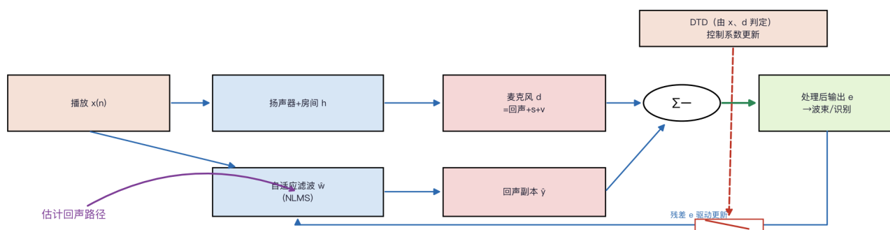
图27 AEC 结构: 根据播放参考估计回声, 再从麦克风信号中相减
