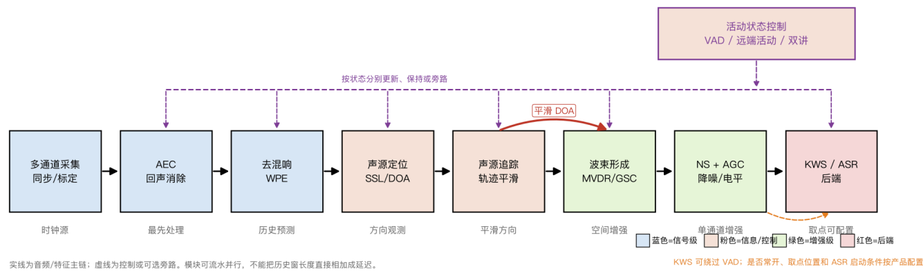
图23 远场语音前端：音频主链、方向反馈、状态控制与可选旁路
