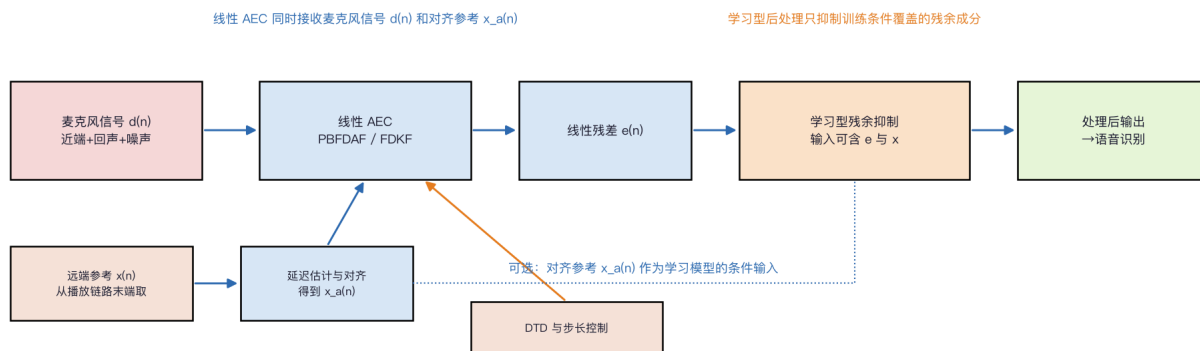
图32 线性回声消除与残余抑制：按系统条件选择模块 (a) 一种常见的混合处理流程
