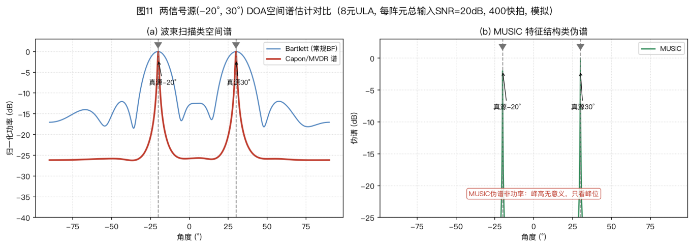
图 11 在同一个两源仿真 (−20°、30°) 中比较 Bartlett、Capon 和 MUSIC。Bartlett 与 Capon 按各自的标准空间谱公式计算；MUSIC 给出伪谱，峰高不是功率。高信噪比 (SNR, signal-to-noise ratio)、快拍 (snapshot, 阵列同一时刻所有麦的一组采样) 充足、源数正确且阵列模型准确时，Capon 和 MUSIC 的窄峰才能转化为可靠的分辨率优势。
