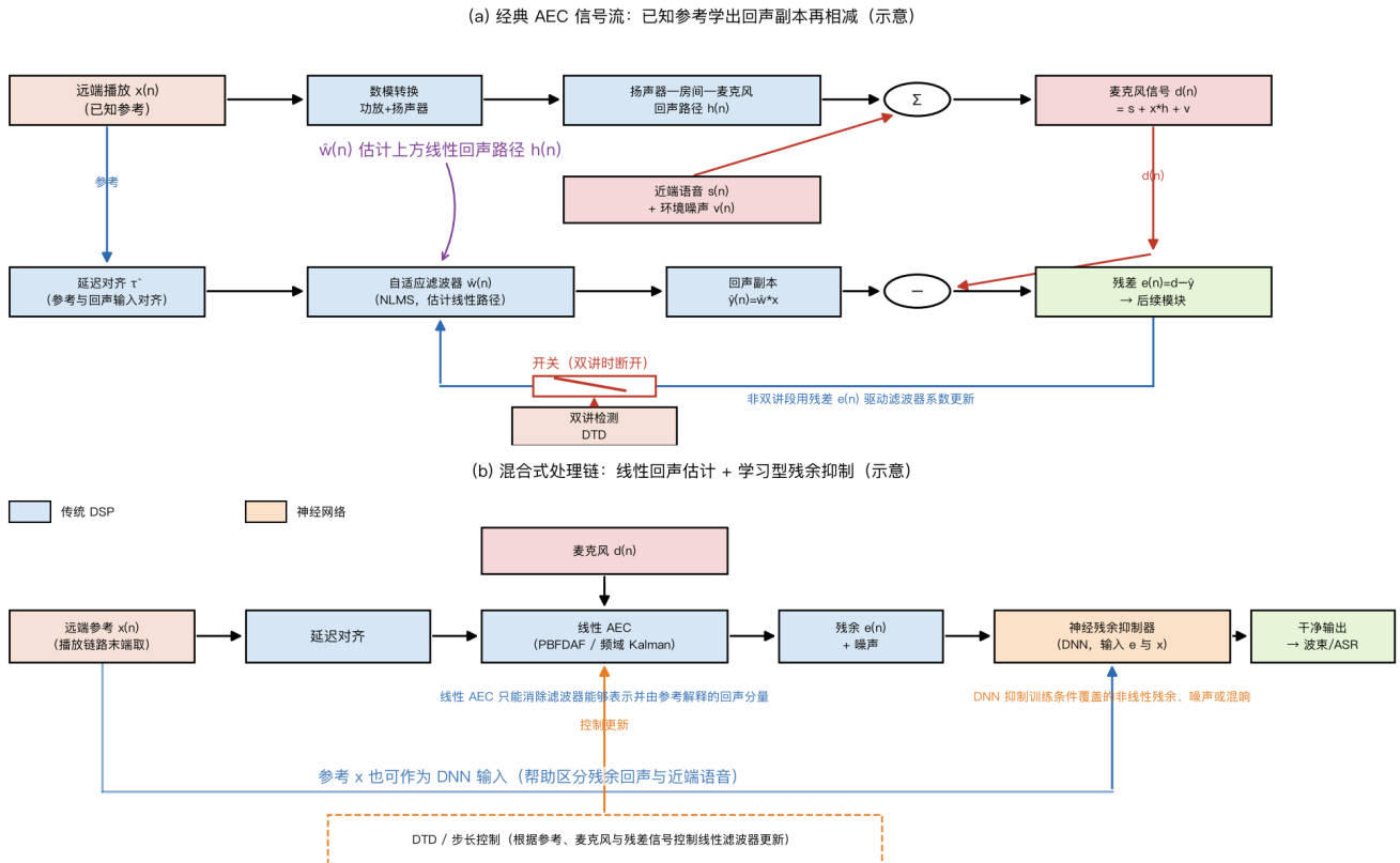
图20 AEC 信号处理链：自适应滤波与混合式结构（示意）
