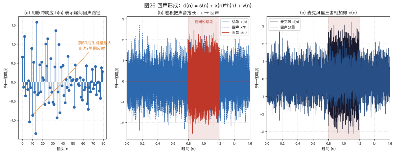
图26 (a) 用冲激响应 h(n) 表示房间路径，前部主要包含直达声和早期反射，后部是逐渐衰减的拖尾。(b) 给出远端参考、卷积后的回声和 0.8~1.2 s 的近端语音。(c) 显示三者在麦克风信号 d(n) 中叠加。AEC 根据参考估计回声分量，再从 d(n) 中减去该估计。
