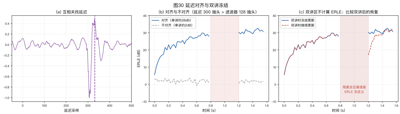
图30 (a) 用互相关估计参考与麦克风信号之间的延迟, 本例峰值约为 331 个采样, 其中包含设置的 300 个采样纯延迟和回声路径主峰的位置。(b) 对齐后的远端单讲 ERLE 约为 28 dB, 不对齐时约为 2 dB。本例的纯延迟超过 128 抽头滤波器的覆盖范围, 因此差异较大。(c) 比较双讲期间冻结和继续更新; 后者会使路径估计偏离, 双讲结束后需要重新收敛。排查时应分别检查延迟估计和双讲控制。
