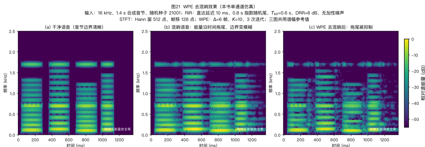
图21 的横轴约为 0~1400 ms，纵轴约为 0~2.5 kHz，颜色表示相对能量的 dB 值。(a) 给出无混响参考；(b) 加入合成混响后，音节结束处出现横向拖尾；(c) 经本书单通道 WPE 示例处理后，拖尾减弱，但仍有残留。该图用于观察同一示例的前后差异，不代表公开数据集上的平均性能。
