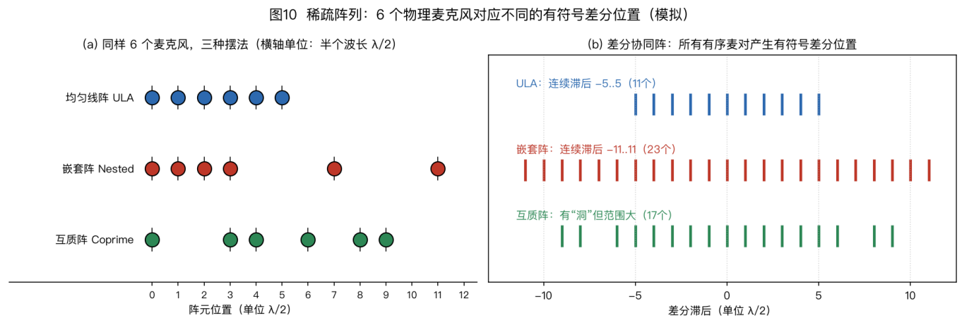
图 10 左侧比较均匀、嵌套和互质三种摆法，横轴单位是半波长；右侧枚举所有有序麦对的位置差，得到有符号差分位置（也称有符号滞后）。均匀阵有 11 个连续滞后，图中的嵌套阵有 23 个连续滞后，互质阵覆盖范围更大但中间有空缺。连续滞后数描述虚拟孔径结构，不应直接写成 MUSIC 可分辨的源数。
