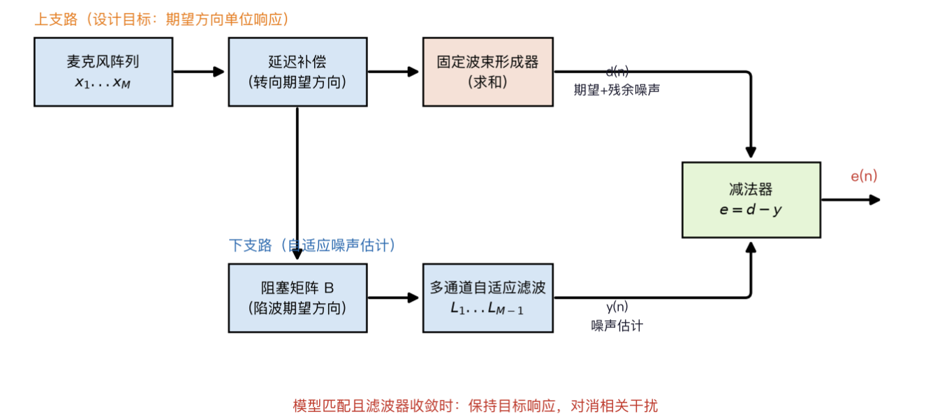
图17 GSC（广义旁瓣对消器）结构框图
