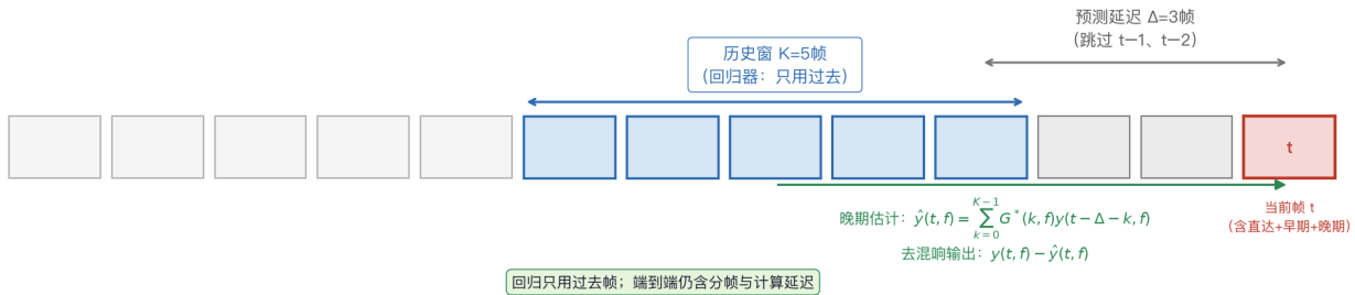
图24 WPE 延迟预测： \Delta=3 时保护 t-1 、 t-2 ， K=5 使用 t-3 \dots t-7
