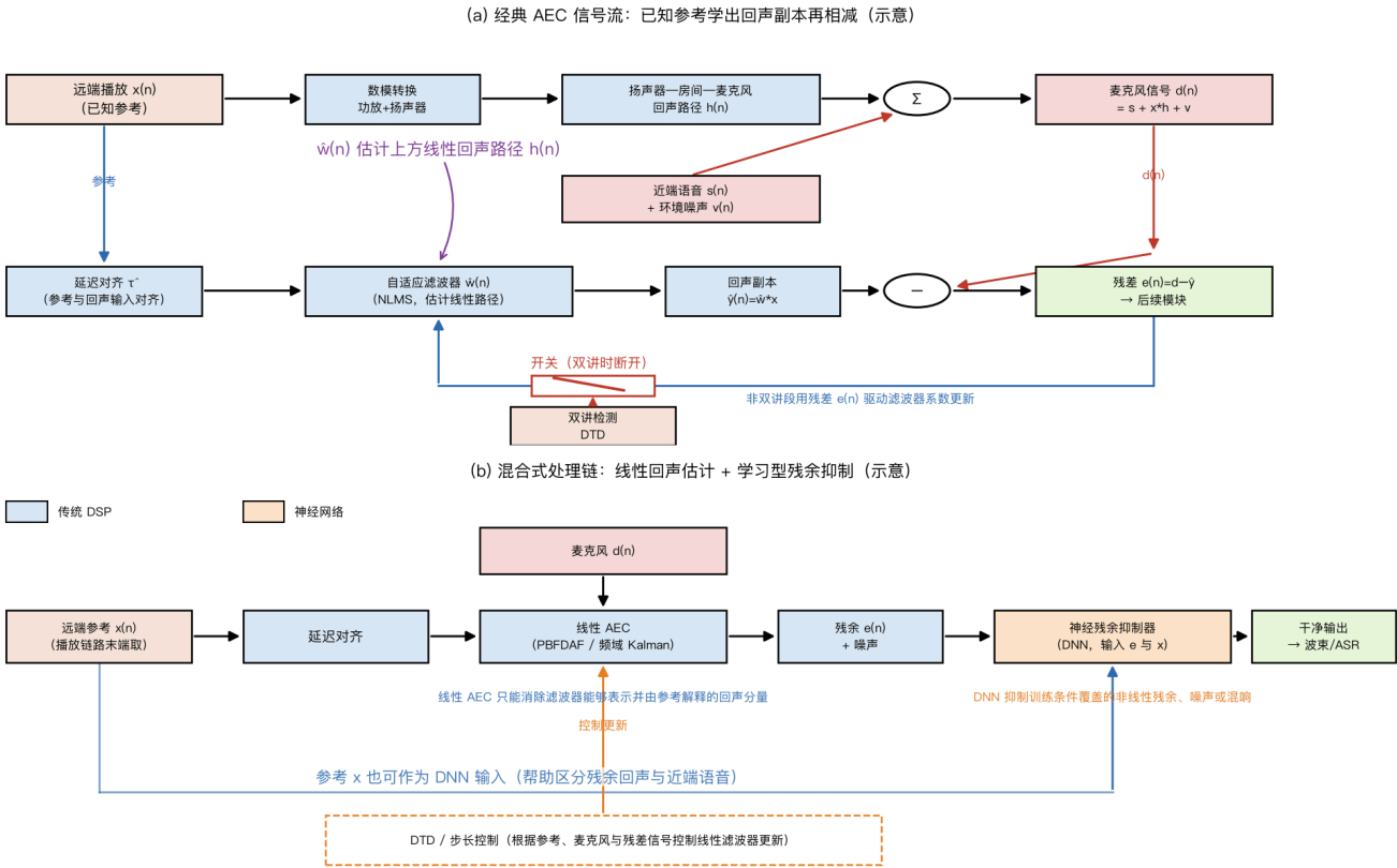
图20 AEC 信号处理链: 自适应滤波与混合式结构 (示意)
