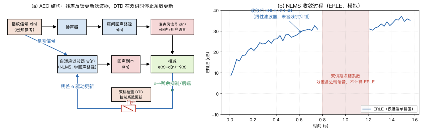
图18 (a) 给出整体结构；(b) 给出 NLMS 在模拟回声路径上的收敛曲线。仿真取 \mu = 0.5 ，回归向量按 \vec{x}(n) = [x(n), x(n-1), \dots, x(n-L+1)]^\top 排列，与生成回声的卷积索引一致，不额外引入一拍延迟。图中标注的是固定随机种子下 0.45 < t < 0.8 s 远端单讲窗口的 ERLE 均值；粉色区域表示双讲期间冻结更新，该区间不统计 ERLE。
