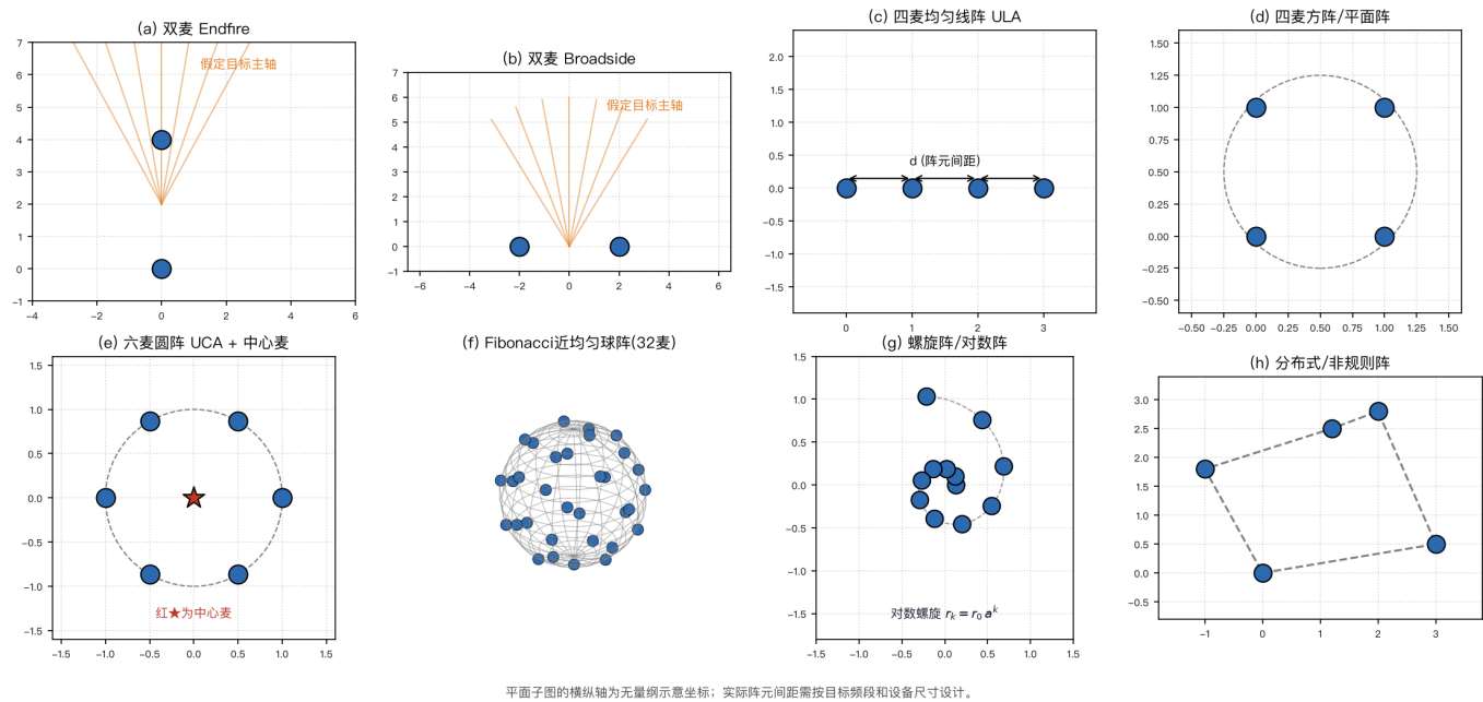
图8 画出八种常见形态：（a）双麦前后排（Endfire）、（b）双麦左右排（Broadside）、（c）四麦均匀线阵、（d）四麦方阵、（e）六麦圆阵加中心麦、（f）按斐波那契球面（Fibonacci sphere）规则确定性布置的 32 麦近均匀球阵、（g）螺旋或对数阵、（h）分布式或非规则阵。（a）（b）的橙色射线表示采用相应波束形成器后的目标主轴：裸露的全向麦克风只有几何位置，不会仅凭摆成前后或左右排列就产生主瓣。（d）的四只麦虽然也落在同一个圆周上，这里按方阵的平面几何分析。
