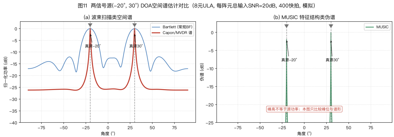
图 11 在同一个两源仿真 (−20°、30°) 中比较 Bartlett、Capon 和 MUSIC。条件为 8 元半波长 ULA、每阵元总输入 SNR 20 dB、400 个快拍，两源相隔 50°；这个较容易的条件只展示三种谱形，不检验最小可分辨角度。Bartlett 与 Capon 按各自的标准空间谱公式计算；MUSIC 给出伪谱，峰高不是功率。只有在源间隔、信噪比、快拍数、源数和阵列失配都明确时，才能用重复试验比较分辨成功率。
