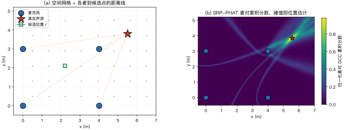
图14 SRP-PHAT 定位过程（独立米级分布式阵列例） 4 m × 3 m 四麦；源(5.5, 3.8) m；c=343 m/s；高斯峰 \sigma=166.7 \mu\text{s} ；90×68网格
