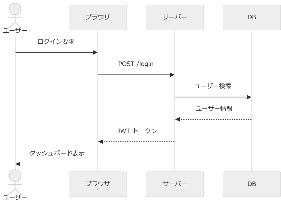
図5.2 ログイン処理のシーケンス図
