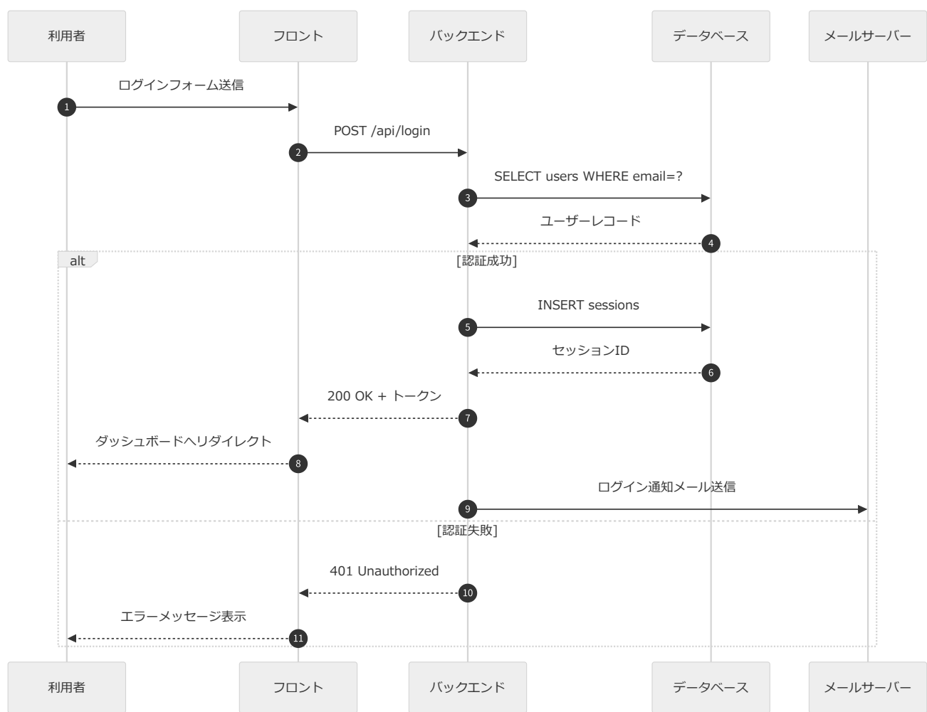
図1.5 フロー図5 ログインシーケンス
