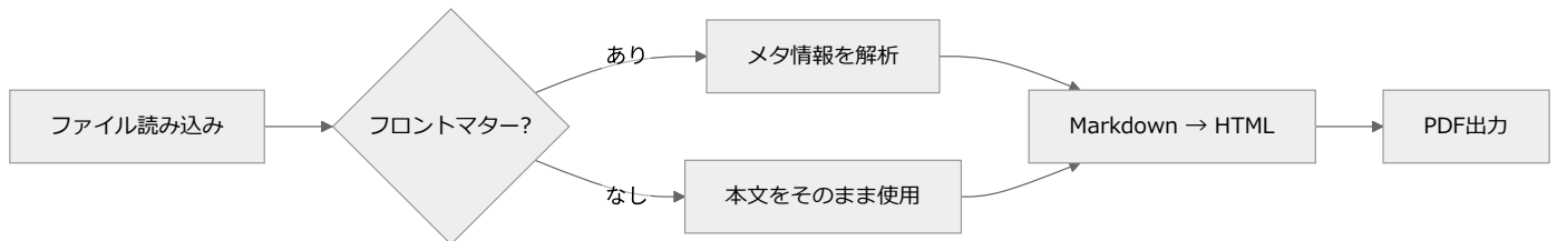
図5.1 Markdown変換パイプラインのフローチャート
