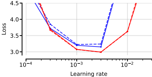
FineWebEdu
