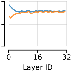
WikiText
