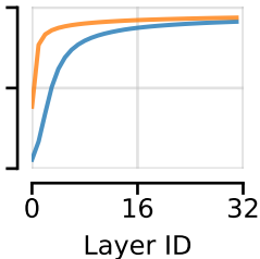
WikiText
