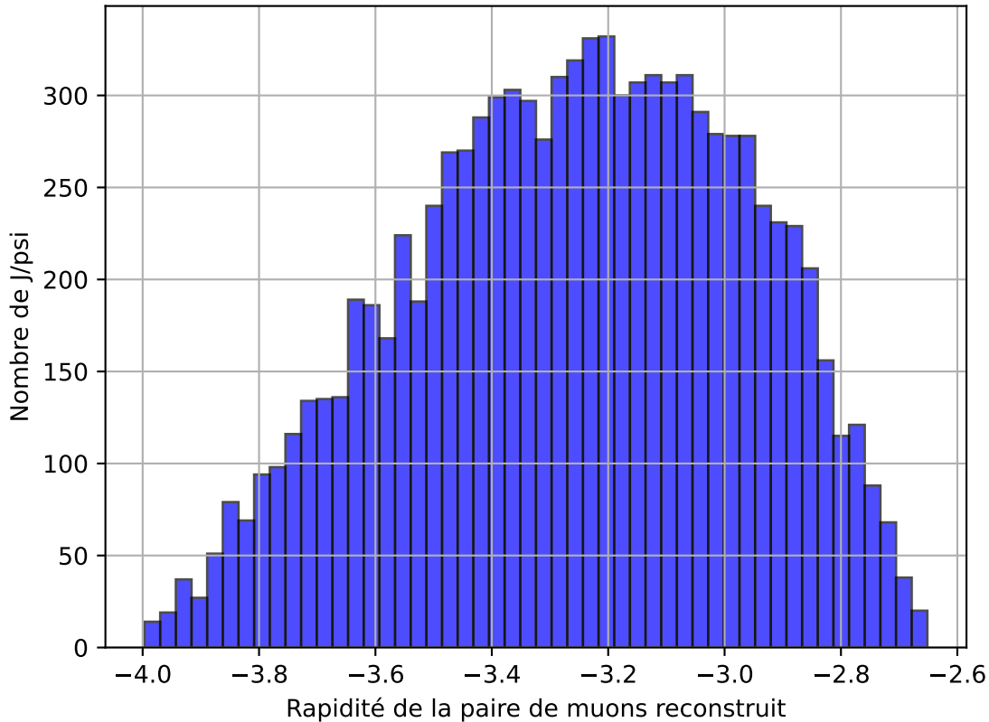
Distribution de la rapidité des paires de muons reconstruit
