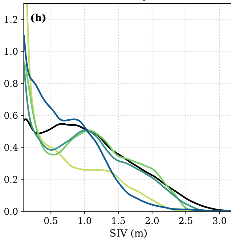
Summer (JAS)
