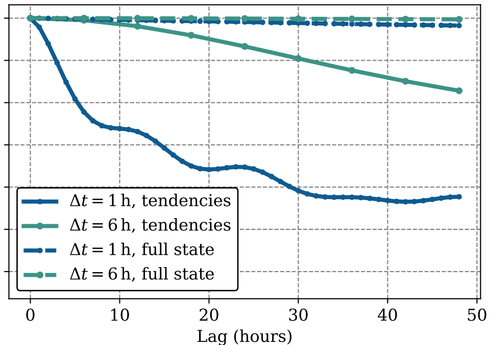
SIV
