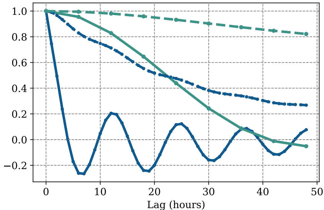
SID
