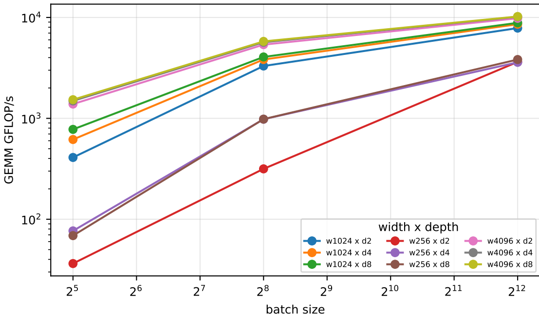
W4 sweep - cudann/nvcc/cublas @ NVIDIA GeForce GTX 1080 Ti (float)
