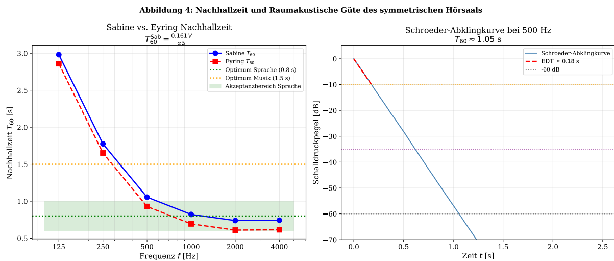
Abbildung 4: Nachhallzeitanalyse des symmetrischen Hörsaals.
