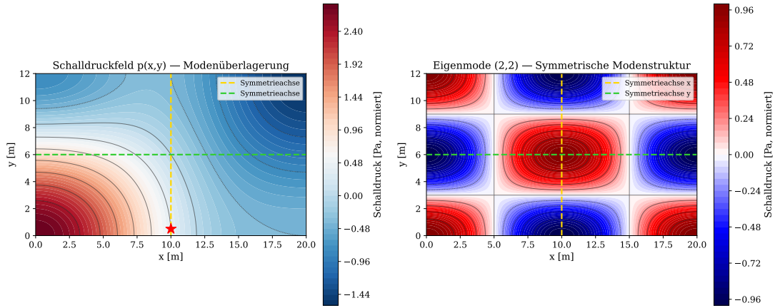
Abbildung 1: Schalldruckfeld im symmetrischen Hörsaal als Draufsicht bei z = 0 .
