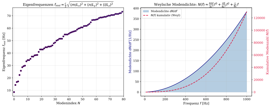
Abbildung 2: Eigenfrequenzstruktur und Weylsche Modendichte des Hörsaals.
