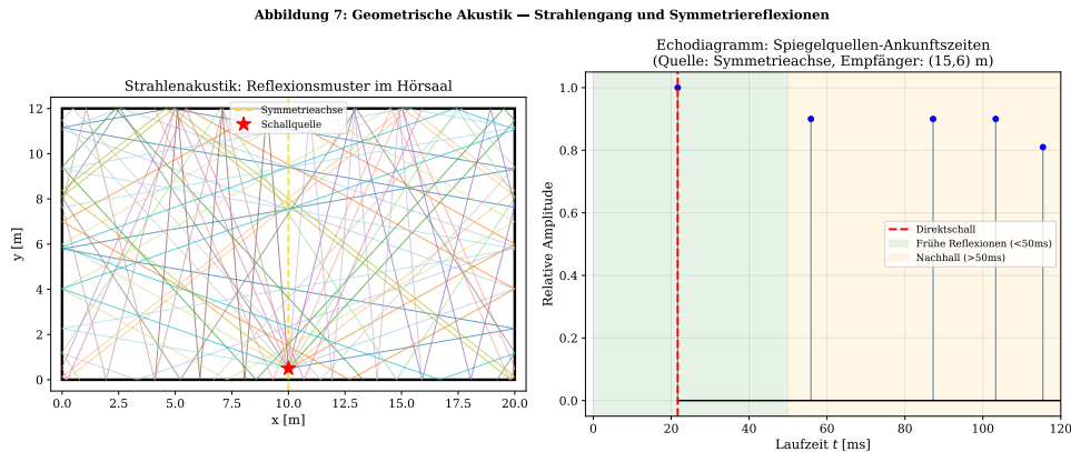
Abbildung 7: Geometrische Akustik des symmetrischen Hörsaals.
