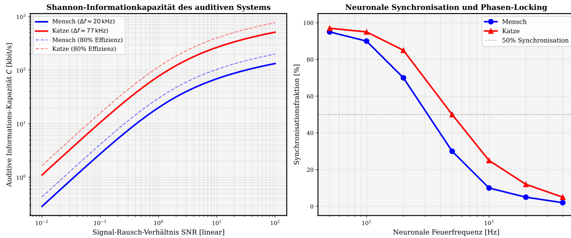
Abbildung 12: Auditive Informationskapazität und neuronale Synchronisation. Linke Tafel: Nach Shannon's Kanalkodierungstheorie (Gl. 22) hat die Katze eine höhere verfügbare Bandbreite und damit eine größere theoretische Informationskapazität für auditive Reizverarbeitung. Rechte Tafel: Die Neuronale Synchronisationsfraktion (phase-locking) zeigt die Fähigkeit von Hörneuronen, synchron mit einem periodischen Stimulus zu feuern. Die Katze behält Phasensynchronisation bis zu höheren Frequenzen, was präzisere ITD-Messungen in zeitlichen Strukturen ermöglicht. Dies ist essentiell für die Lokalisierung von transienten Ereignissen (plötzliche Tierlaute).
