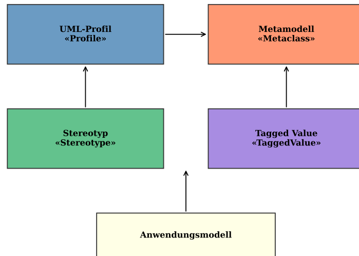
Abbildung 18.1: Struktur eines UML-Profiles mit Zeit-Annotationen
