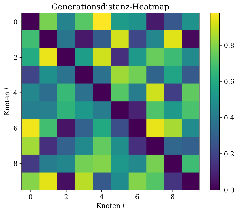
Abbildung 21.10: Generationsdistanz d_{\text{gen}}(A, B) â€“ Heatmap.
