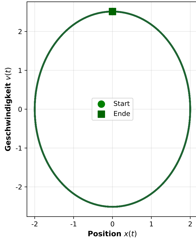
Phasenraum: Gesunde Wirtschaft (Stabiler Grenzzyklus)
