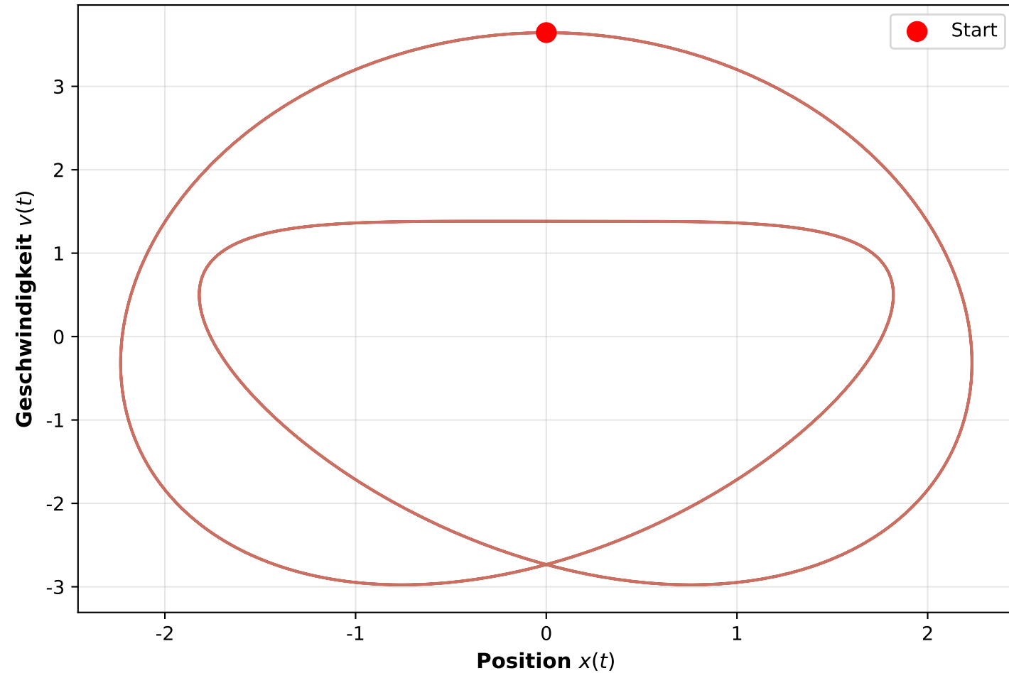
Phasenraum: Kranke Wirtschaft (Chaos durch Überbedarf)
