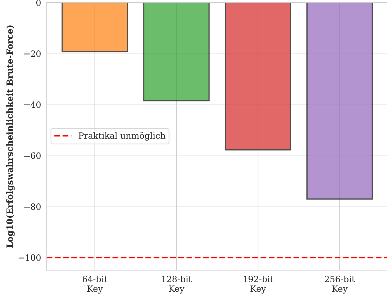
Praktische Unmöglichkeit: Brute-Force Angriffe Gegen informationstheoretisch sichere Systeme
