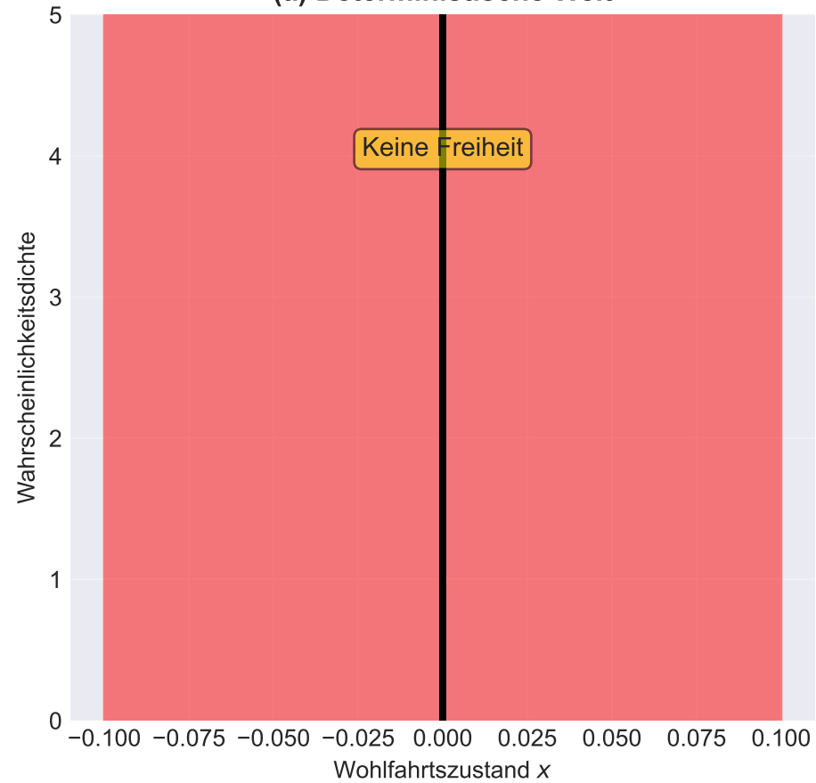
(a) Deterministische Welt
