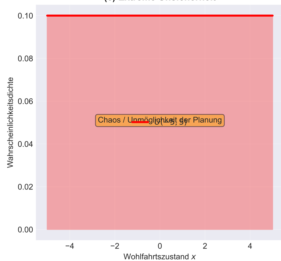
(c) Extreme Unsicherheit
