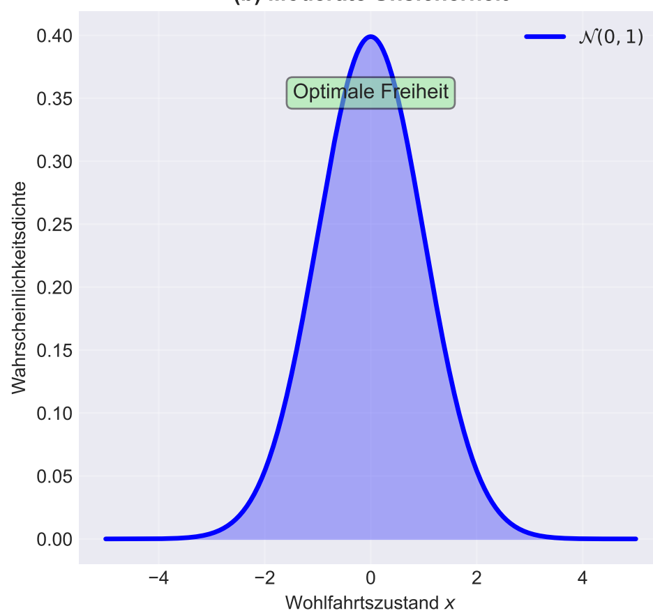
(b) Moderate Unsicherheit
