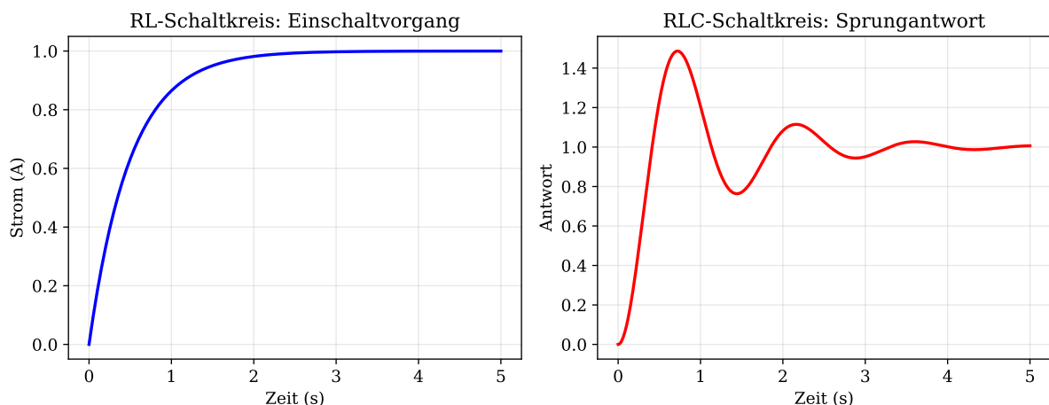
Abbildung 15.3: RL-Stromkreis: Experimentelle Validierung der e-Funktion
