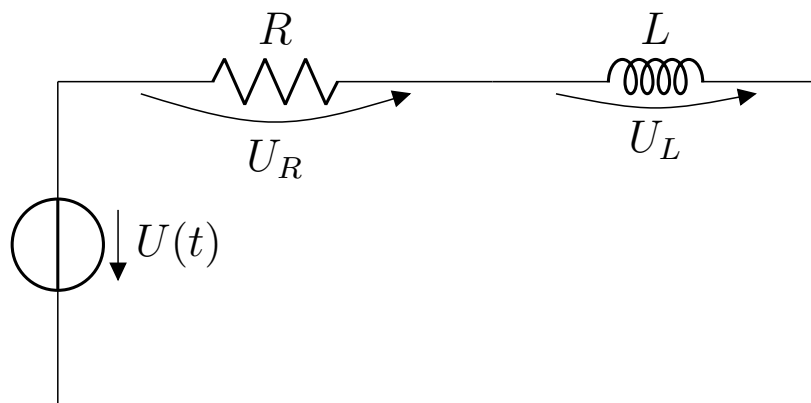
Abbildung 15.1: RL-Stromkreis als Reihenschaltung mit Widerstand R und Induktivität L
