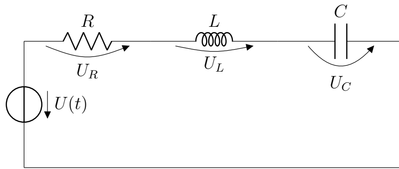
Abbildung 15.2: RLC-Stromkreis mit Widerstand R , Induktivität L und Kondensator C
