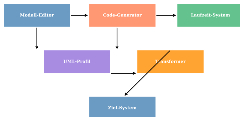
Abbildung 18.3: Zweistufiger Generierungsprozess
