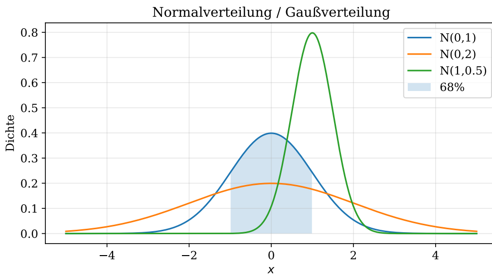
Abbildung 5.3: Gaußsche Verteilung
