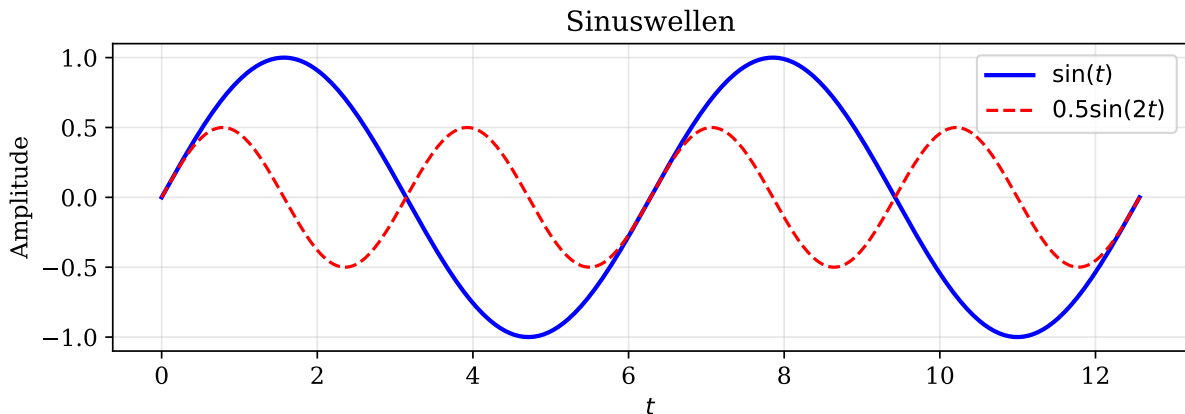
Abbildung 19.2: Sinusschwingung
