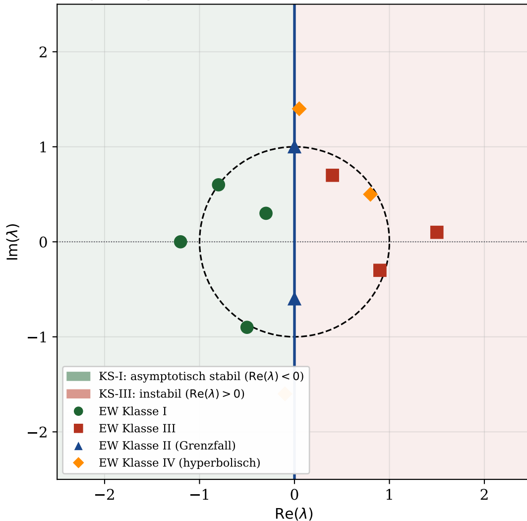
Abbildung 1: Eigenwertraum und Zustandsklassen KS-I bis KS-IV
