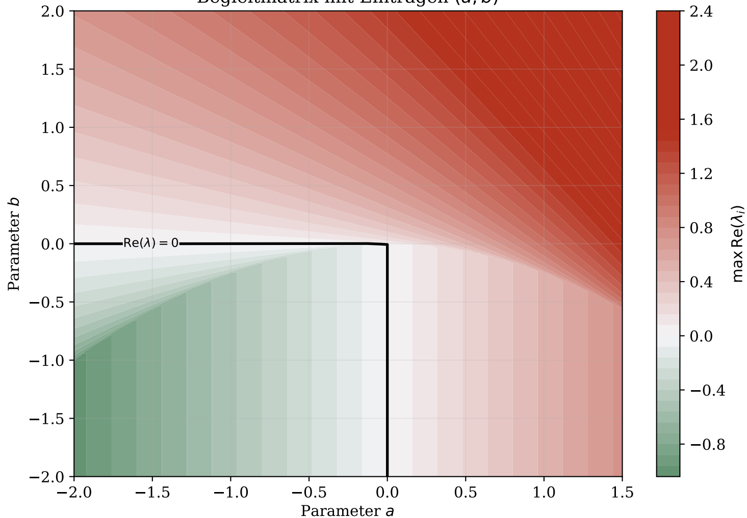
Abbildung 7: Stabilitätskarte – max. Realteil der Eigenwerte Begleitmatrix mit Einträgen (a, b)
