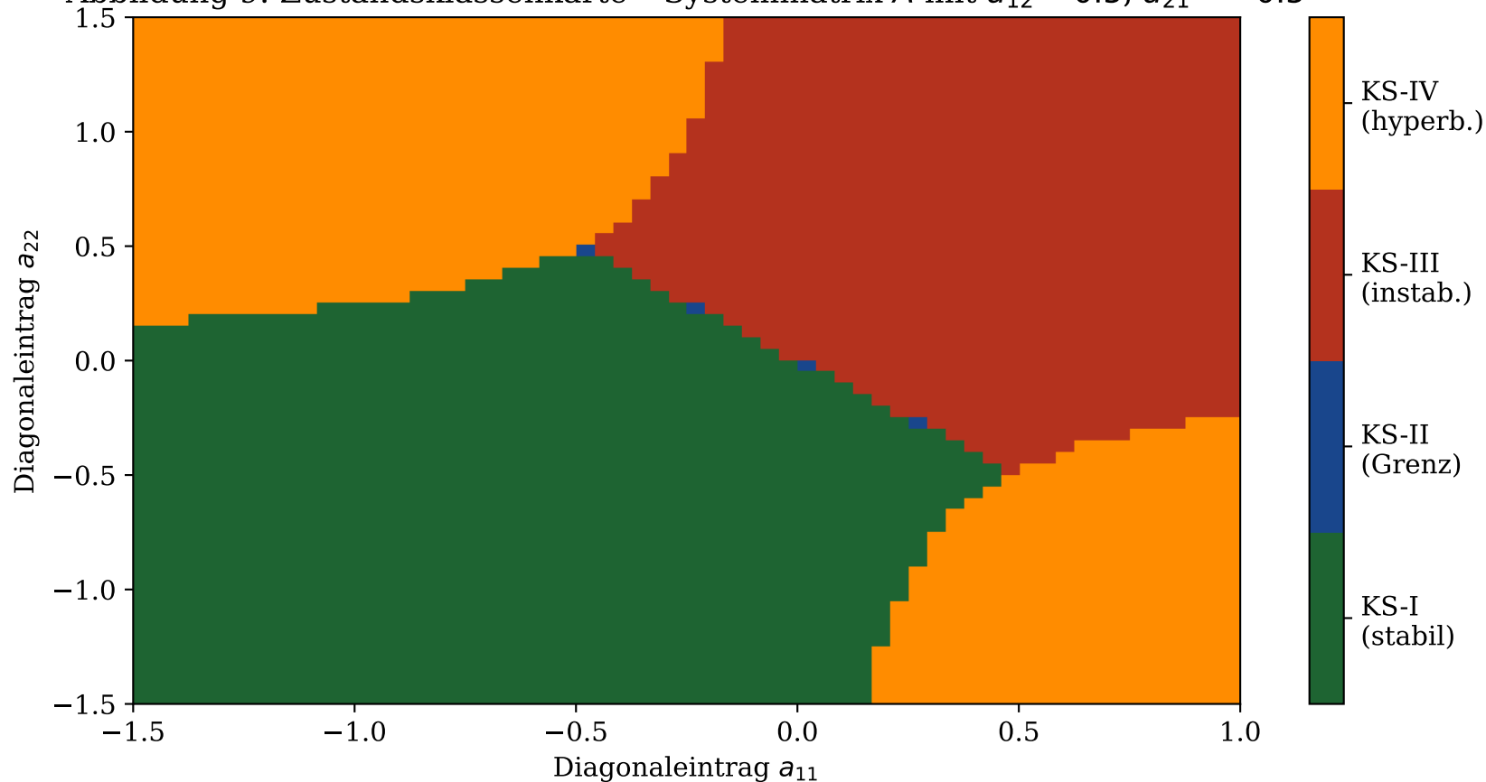
Abbildung 9: Zustandsklassenkarte - Systemmatrix A mit a_{12} = 0.5 , a_{21} = -0.5
