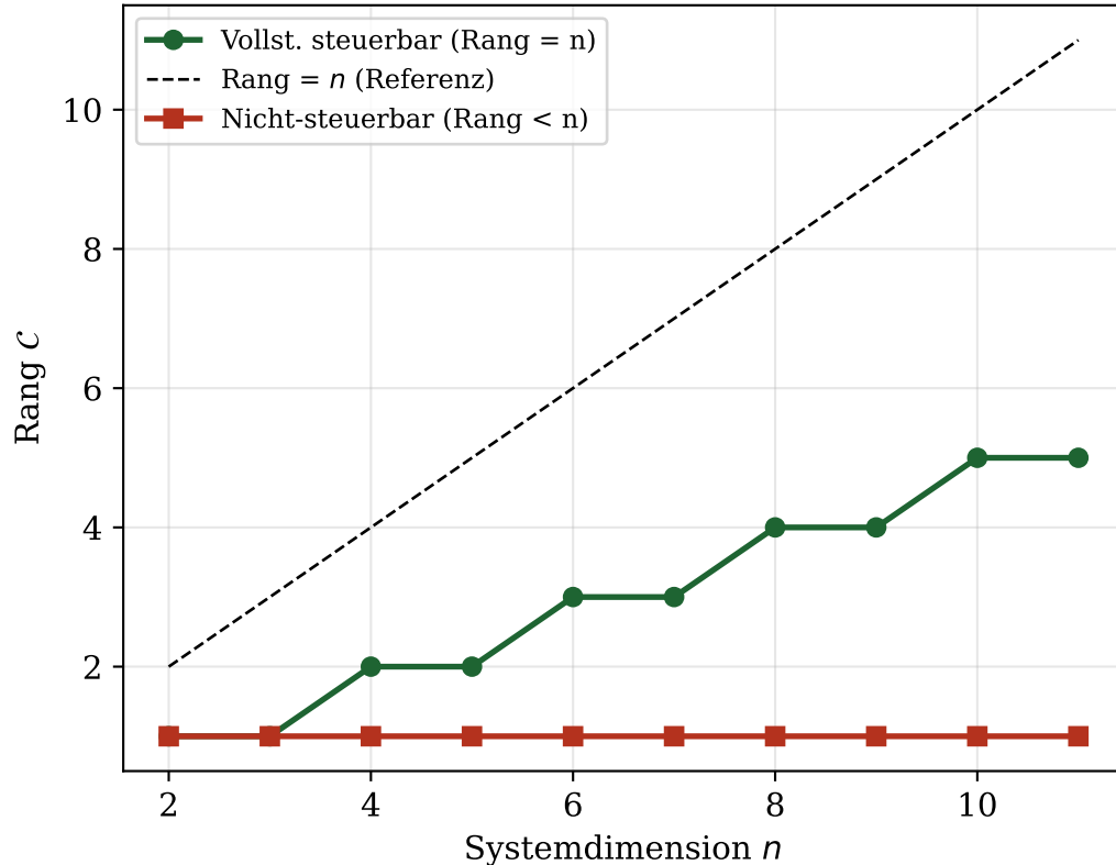
Steuerbarkeitsrang vs. Systemdimension
