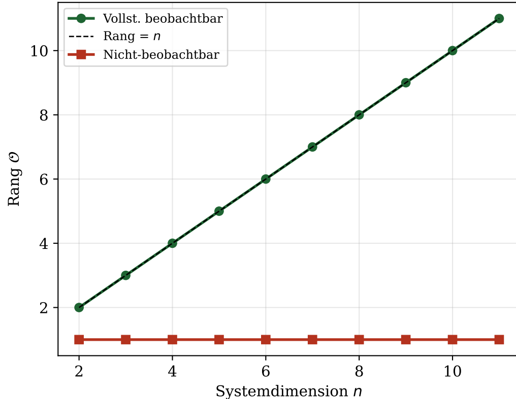
Beobachtbarkeitsrang vs. Systemdimension
