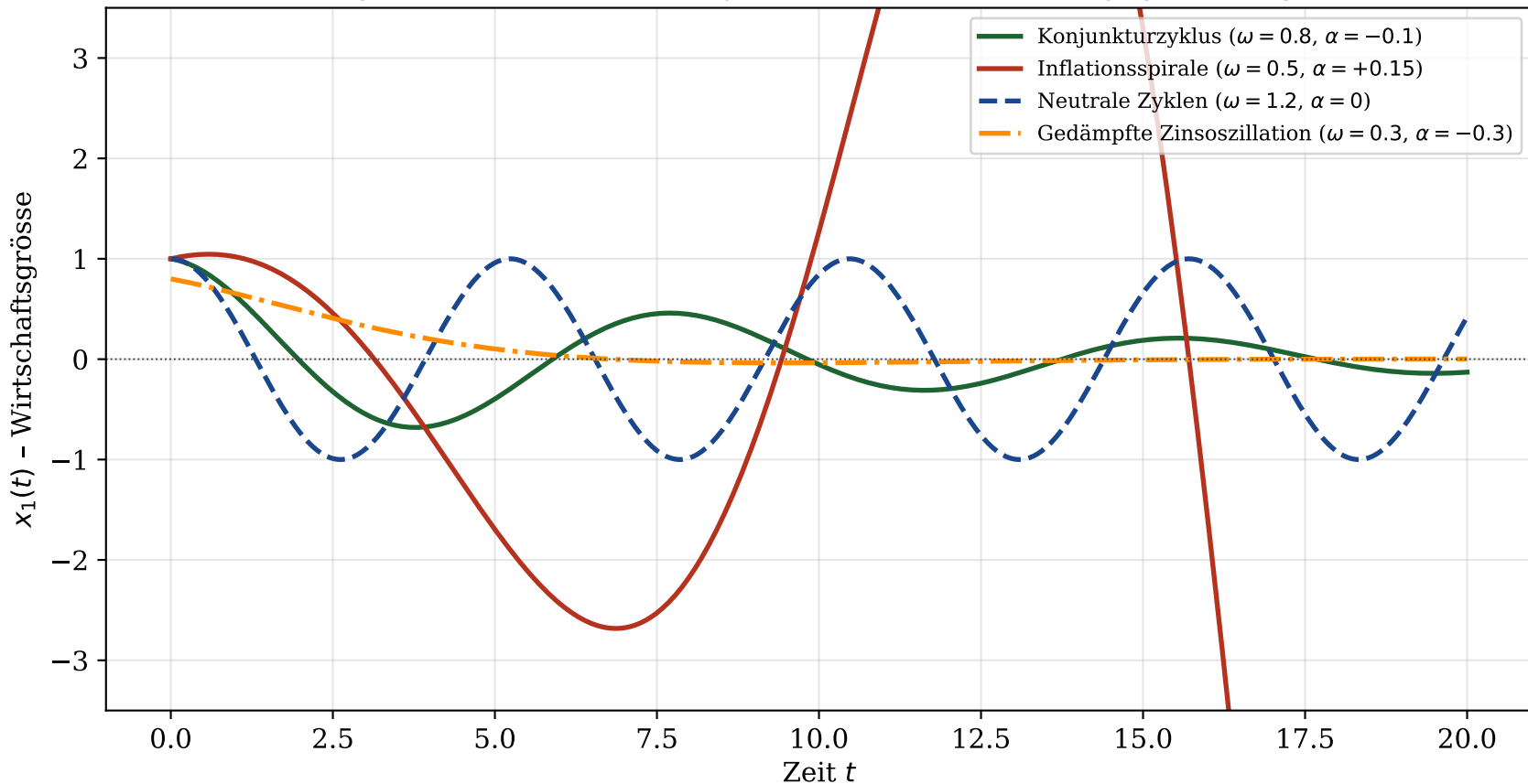
Abbildung 11: Wirtschaftliche Zyklusmodelle durch konjugierte Eigenwerte
