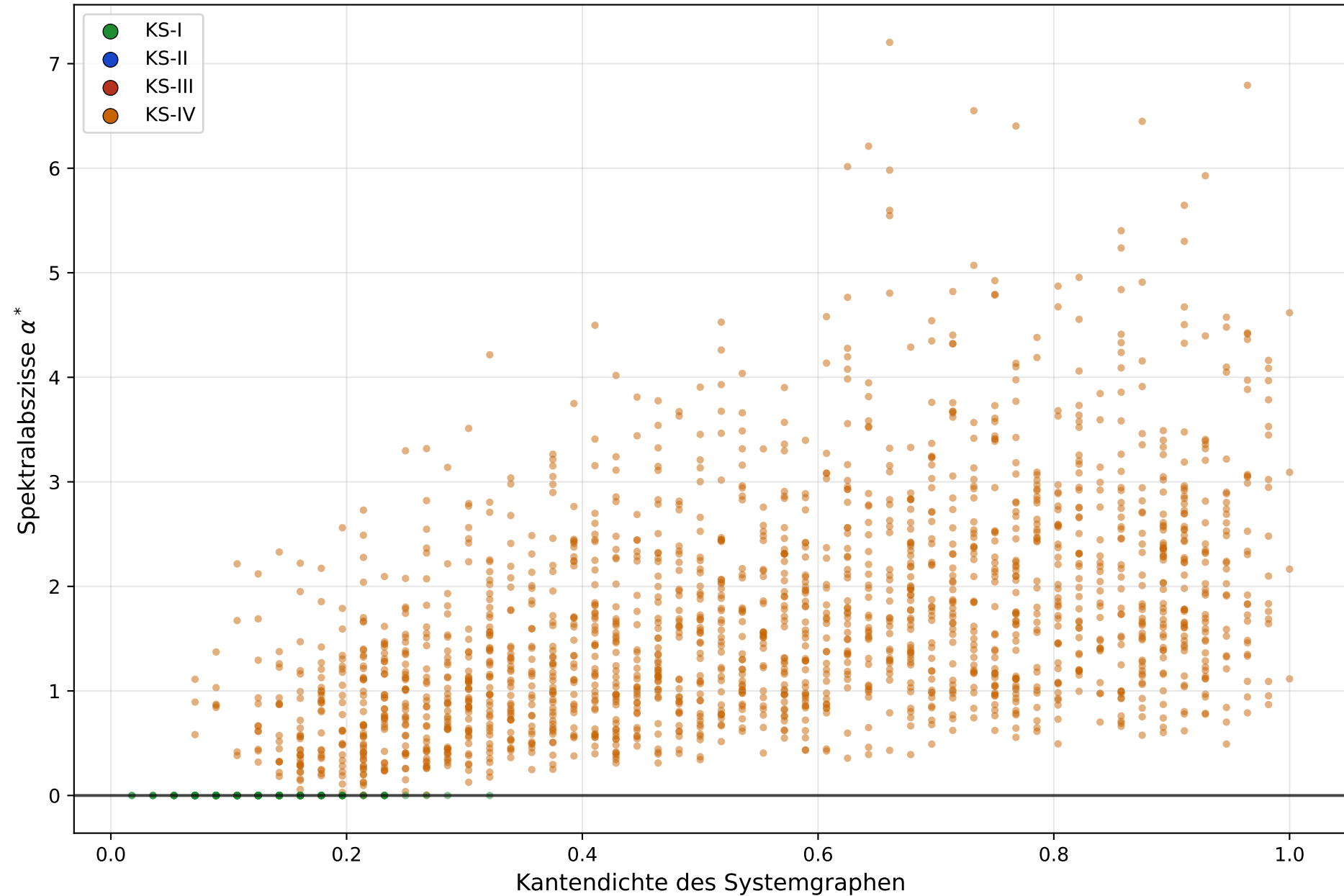
Zustandsklassenkarte: Kantendichte vs. Spektralabszisse
