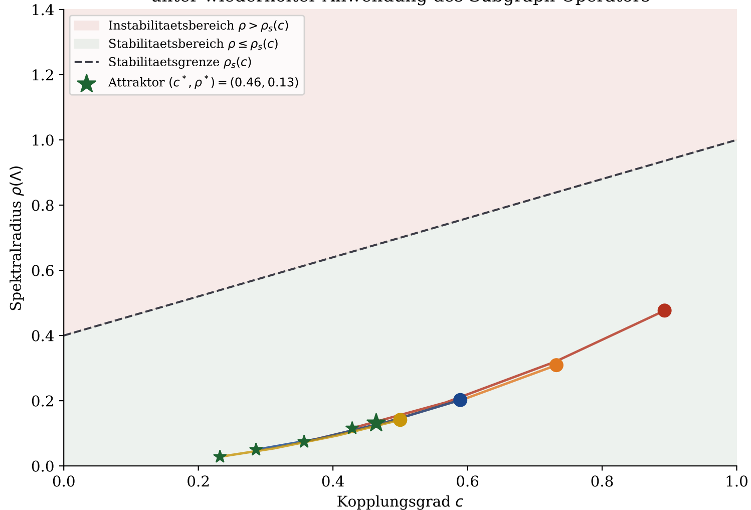
Plot S5 -- Phasendiagramm: Trajektorien im (c, \rho) -Raum unter wiederholter Anwendung des Subgraph-Operators
