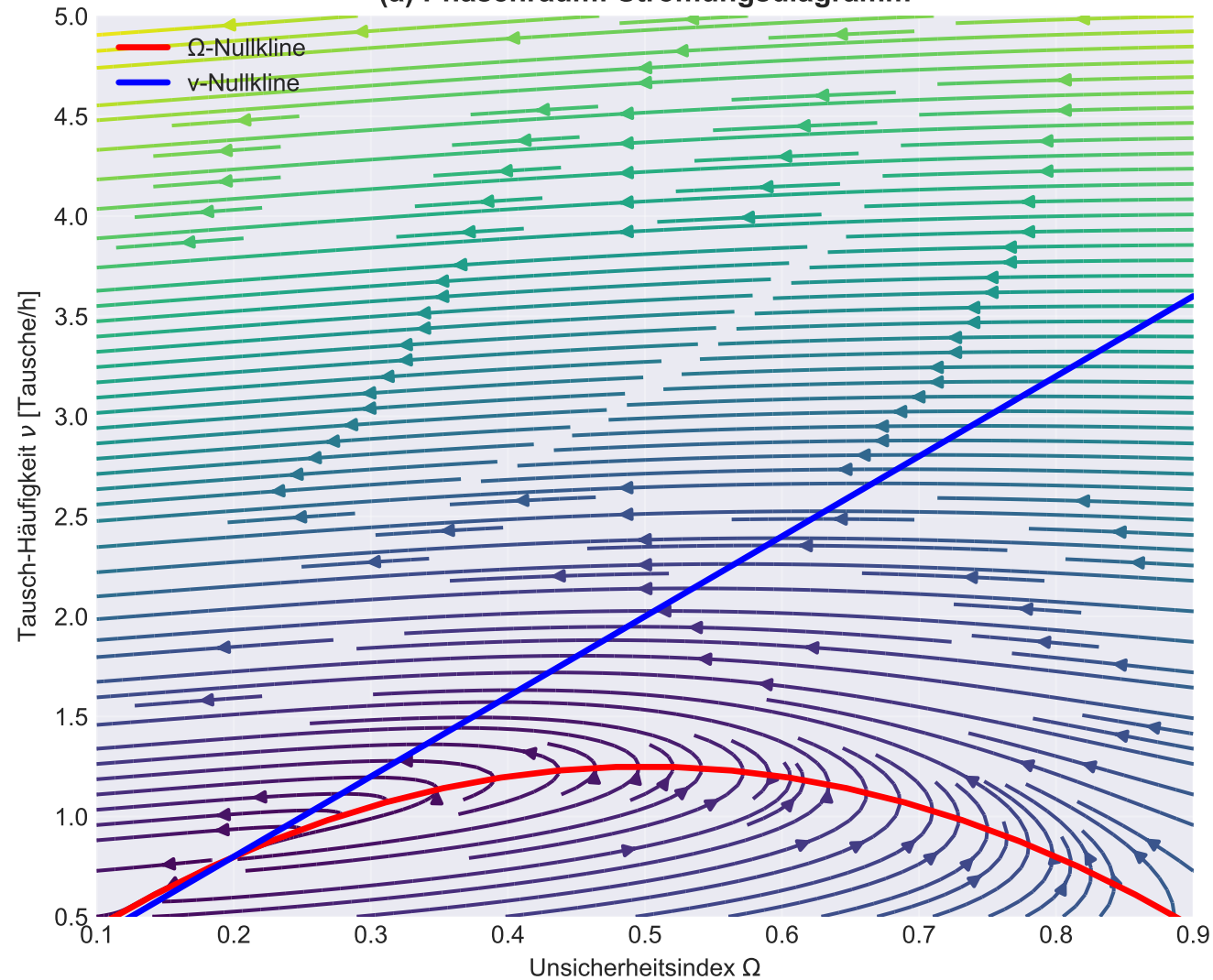
(a) Phasenraum: Strömungsdiagramm
