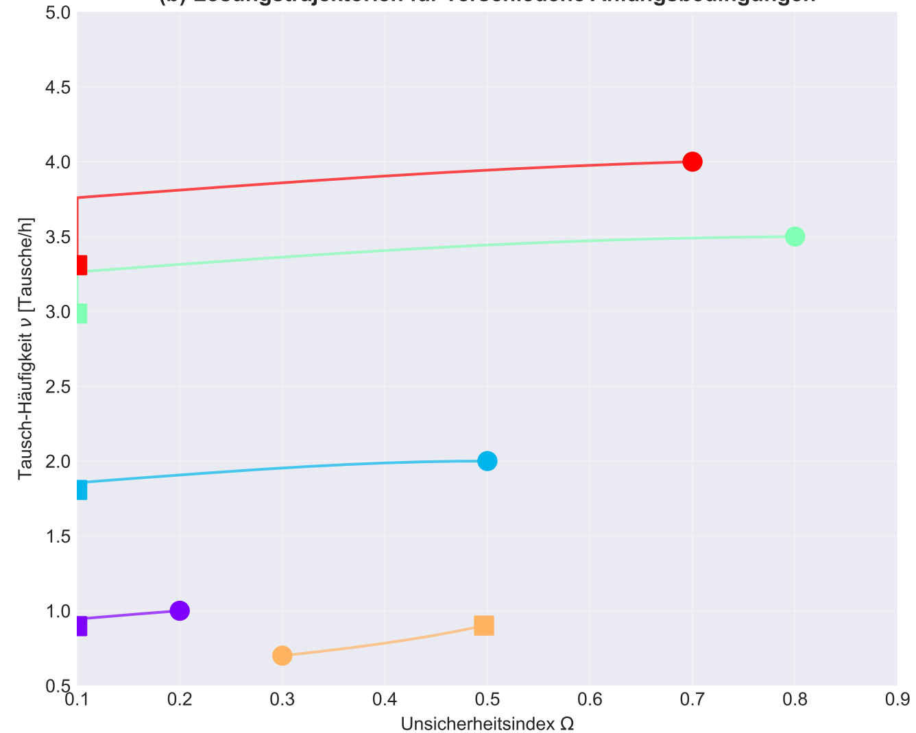
(b) Lösungstrajektorien für verschiedene Anfangsbedingungen
