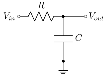
Abbildung 9.1: Der Tiefpassfilter
