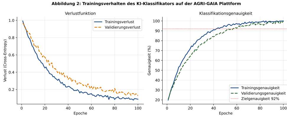
Abbildung 7.2: Trainings- und Validierungsverhalten des KI-Klassifikators über 100 Epochen auf der AGRI-GAIA Plattform. Beide Kurven konvergieren stabil; die Validierungsgenauigkeit überschreitet die Zielmarke von 92 % ab Epoche \approx 68 .
