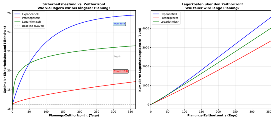
Abbildung 5.3: Optimaler Sicherheitsbestandsmenge als Funktion des Zeithorizonts für verschiedene Degradationsmodelle.
