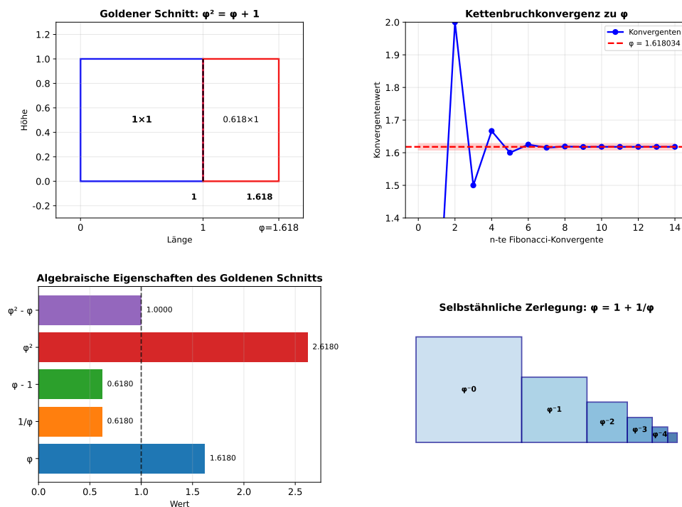
Abbildung 9.2: Der Plot zeigt die geometrische, algebraische und Fibonacci-basierte Struktur des Goldenen Schnitts.
