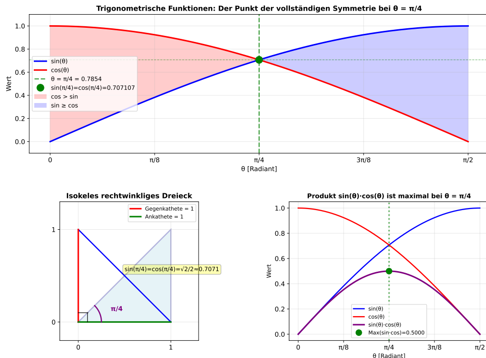
Abbildung 9.3: Der Plot macht den Gleichheitspunkt von Sinus und Kosinus bei \theta = \pi/4 geometrisch und analytisch sichtbar.
