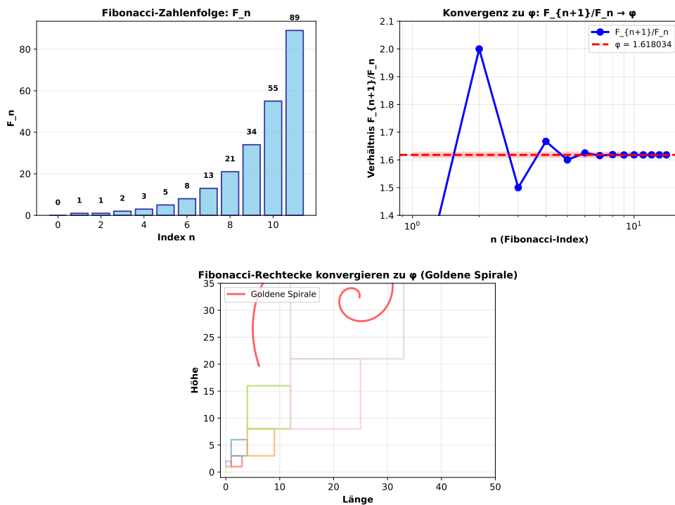
Abbildung 9.5: Der Plot verbindet das Wachstum der Fibonacci-Zahlen, die Quotientenkonvergenz zu \phi und die zugehörige Rechteckkonstruktion.
