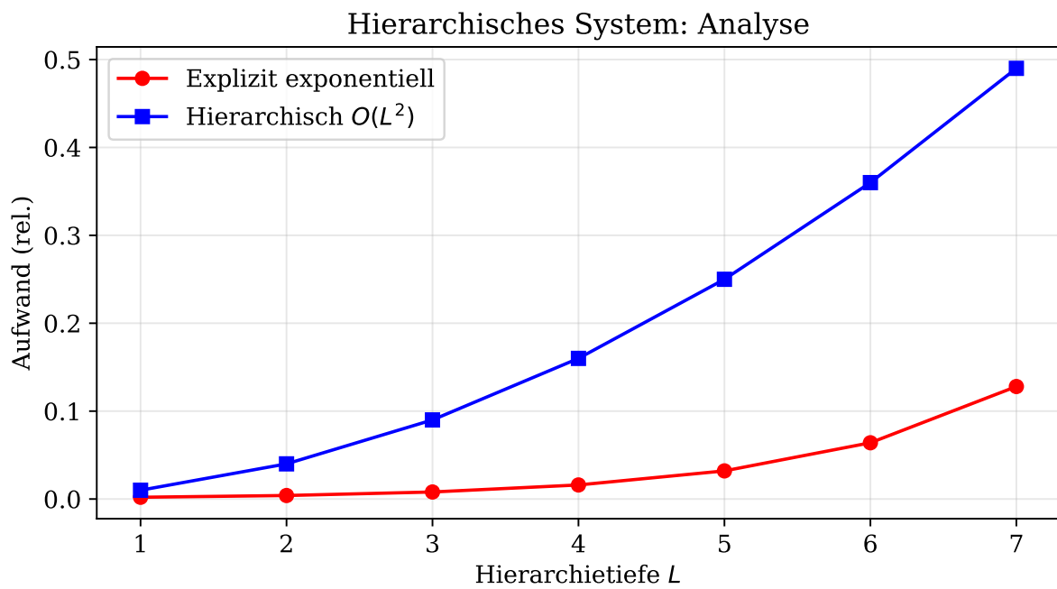
Abbildung 16.9: Experiment 6: Hierarchisches System
