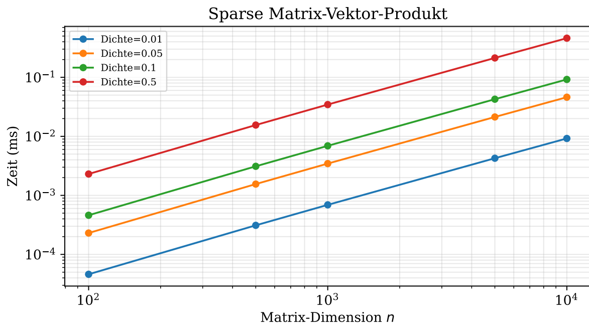
Abbildung 16.5: Experiment 2: Performance sparse Matrix-Vektor-Multiplikation
