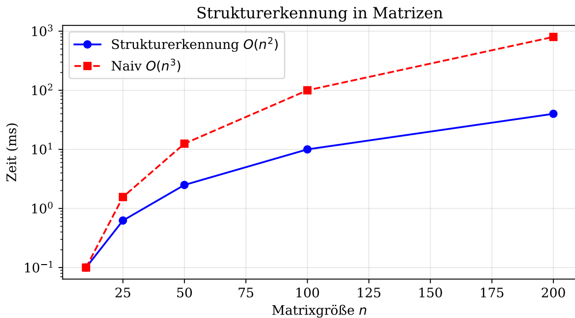
Abbildung 16.7: Experiment 4: Automatische Strukturerkennung
