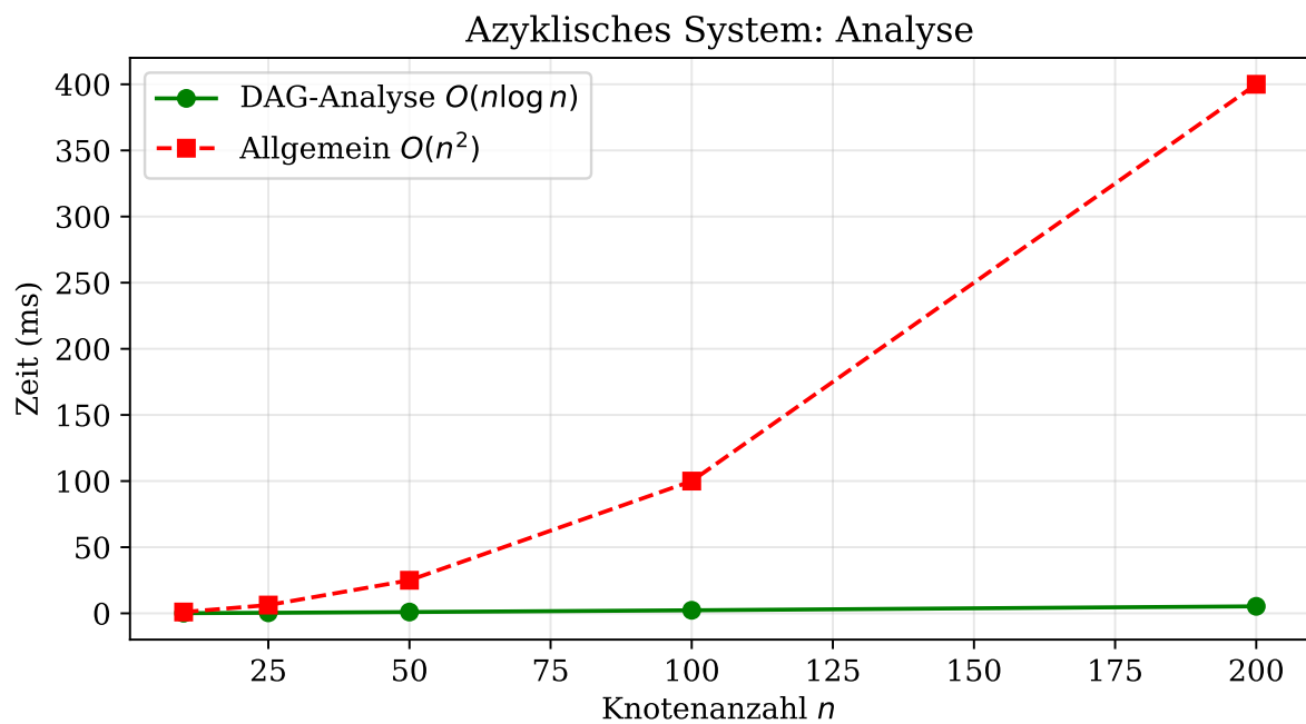
Abbildung 16.10: Experiment 7: Azyklisches System
