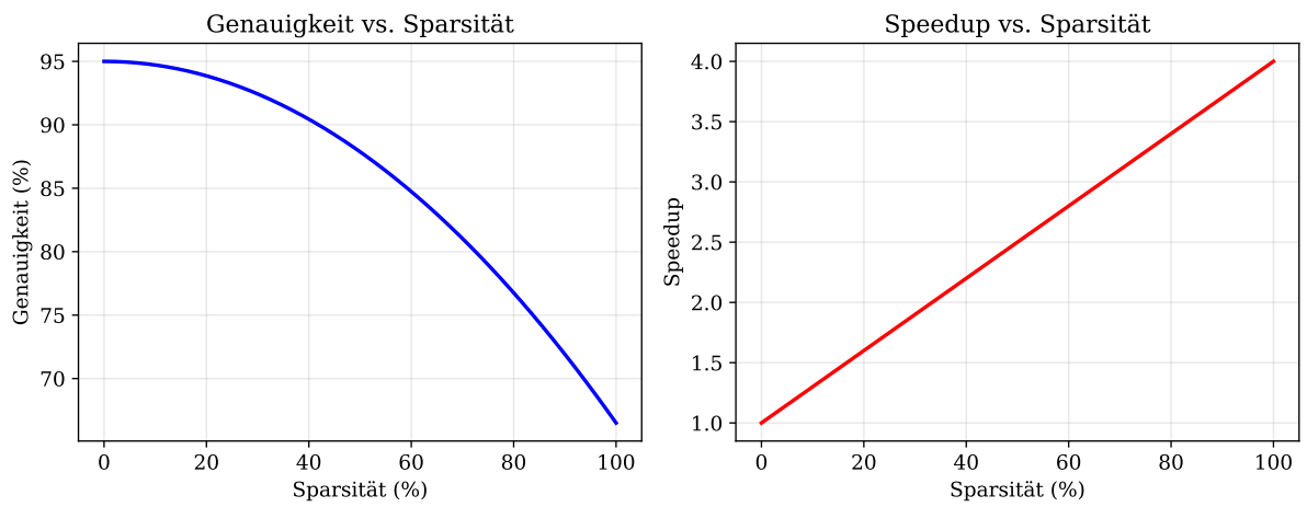
Abbildung 16.6: Experiment 3: Sparsity in neuronalen Netzen
