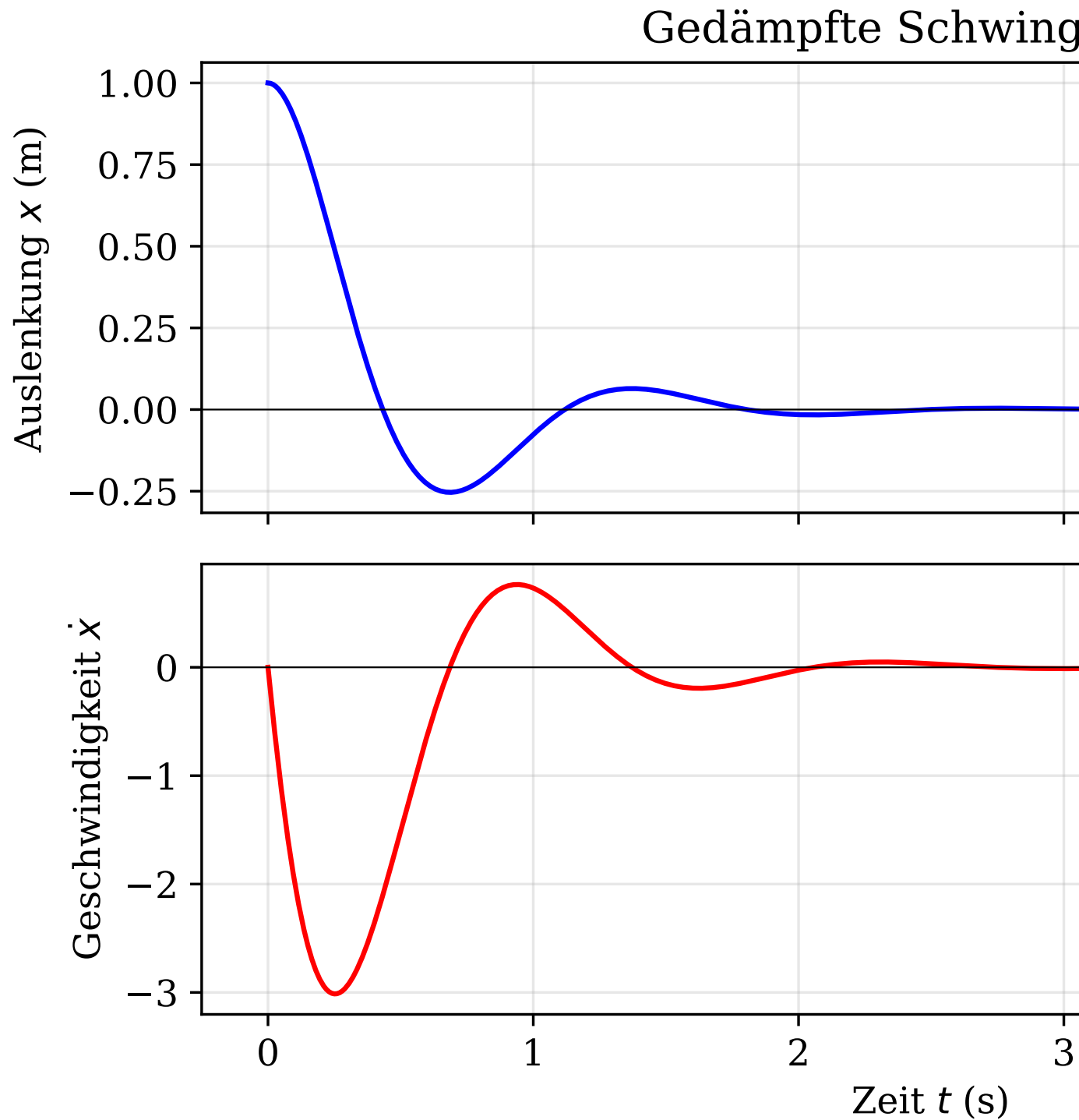
Abbildung 16.3: Zeitliche Entwicklung der Auslenkung: Gedämpfte Schwingungen
