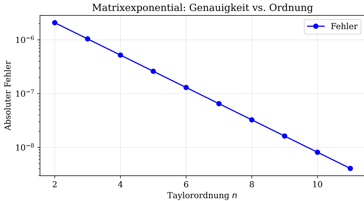
Abbildung 16.4: Experiment 1: Genauigkeit der Matrixexponential-Methoden
