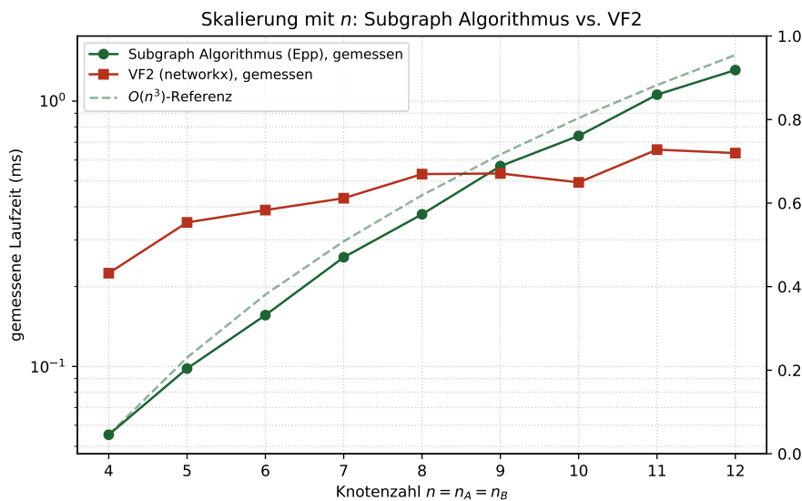
Abbildung 9: Gemessene Laufzeit beider Verfahren bei gemeinsam wachsendem n = n_A = n_B (5 Wiederholungen je n ), zusammen mit einer auf den ersten Messpunkt skalierten O(n^3) -Referenzkurve für den Subgraph Algorithmus.
