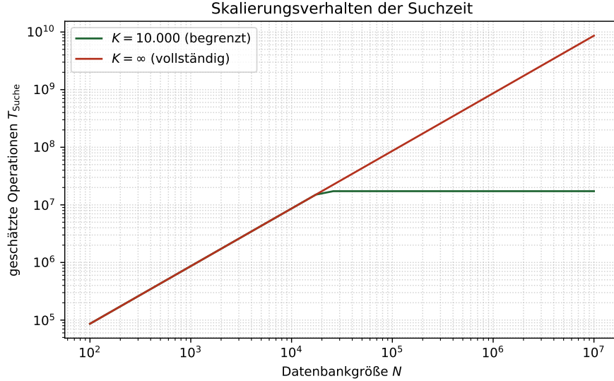
Abbildung 5: Geschätzte Suchzeit T_{\text{Suche}} als Funktion der Datenbankgröße N , für festes Kandidatenlimit K = 10.000 und K = \infty (volle Pipeline), gemäß Satz 2.
