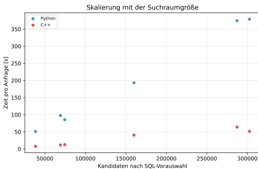
Abbildung 17: Die Antwortzeit nimmt für beide Backends mit der nach der SQL-Vorauswahl verbleibenden Kandidatenzahl zu.
