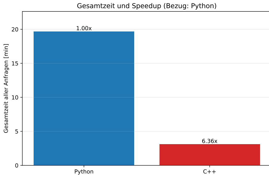
Abbildung 14: Die Gesamtlaufzeit der sechs Suchen sinkt mit der C++-Library gegenüber Python auf rund ein Sechstel.
