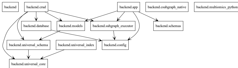
Abbildung 1: UML-Paketdiagramm der Gen-DB-Architektur.
