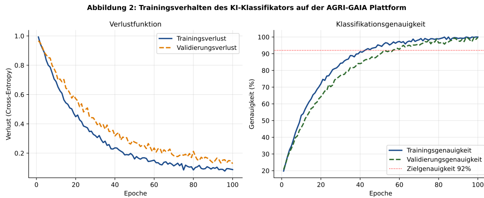
Abbildung 8.2: Trainings- und Validierungsverhalten des KI-Klassifikators über 100 Epochen auf der AGRI-GAIA Plattform. Beide Kurven konvergieren stabil; die Validierungsgenauigkeit überschreitet die Zielmarke von 92 % ab Epoche \approx 68 .
