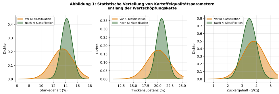
Abbildung 8.1: Statistische Qualitätsparameterverteilungen vor und nach Einführung des KI-Klassifikators. Die signifikante Reduktion der Standardabweichung ( \sigma_{q_1} : 1,8 \rightarrow 0,9 , \sigma_{q_2} : 2,3 \rightarrow 1,1 , \sigma_{q_3} : 0,8 \rightarrow 0,5 ) belegt die verbesserte Qualitätshomogenität.
