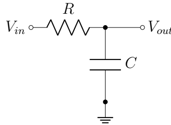
Abbildung 10.1: Der Tiefpassfilter
