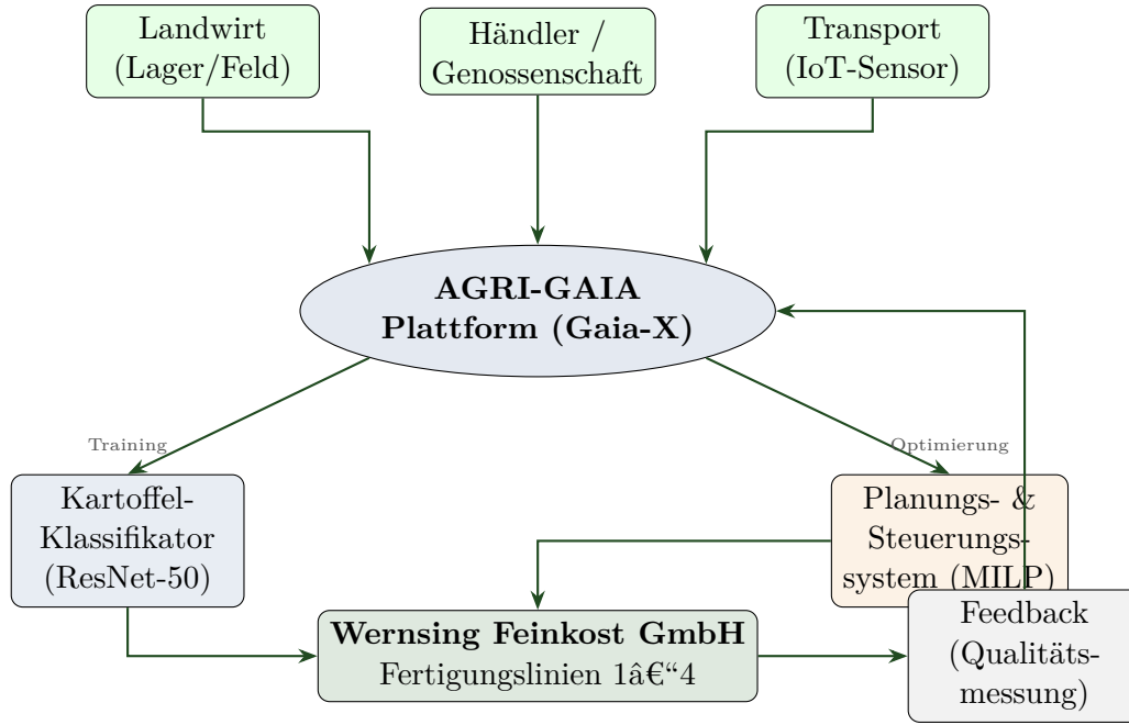
Abbildung 8.3: Systemarchitektur des AGRI-GAIA AP5.3/5.4. Qualitätsdaten fließen von Landwirten, Händlern und Transport-IoT-Sensoren zur zentralen AGRI-GAIA Plattform. Der Klassifikator ermittelt Qualitätsklassen, das Planungssystem optimiert die Rohstoffallokation; beide Module lernen kontinuierlich aus Fertigungsrückmeldungen.
