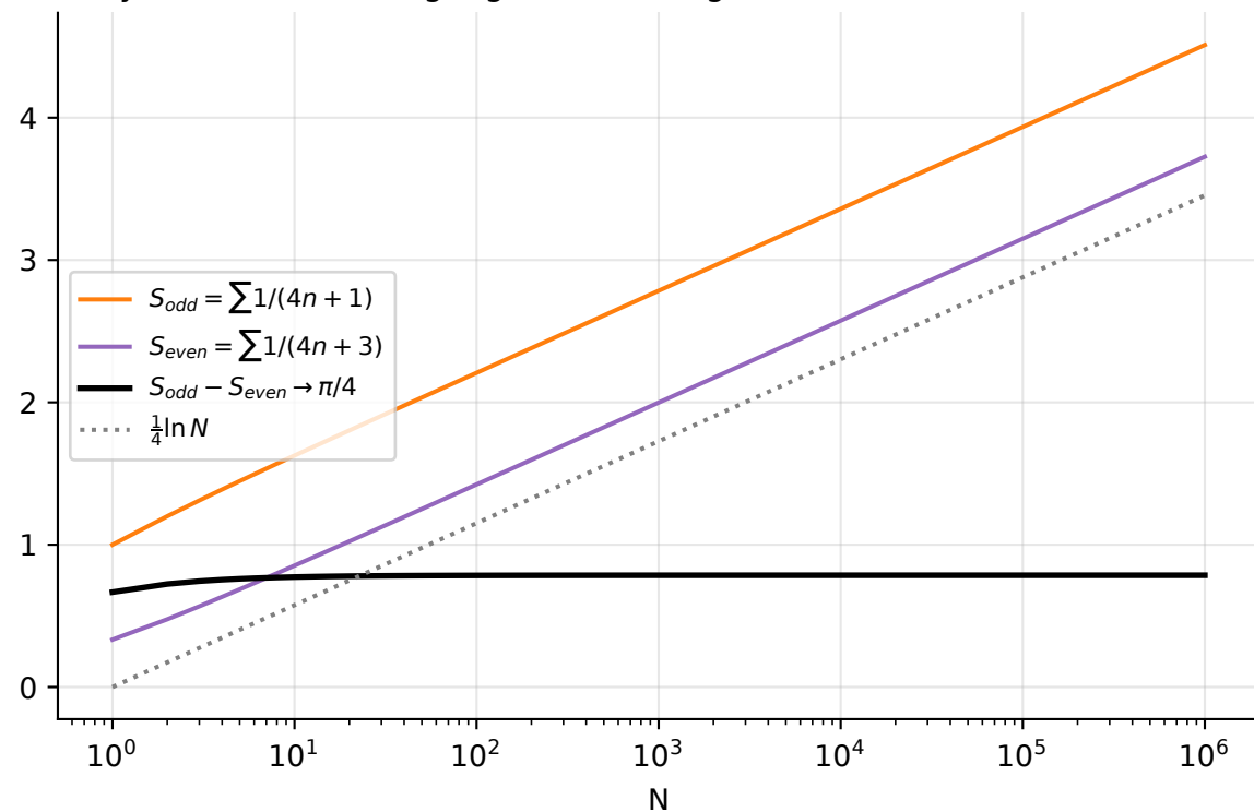
Asymmetrische Zerlegung: beide divergieren ( \sim \frac{1}{4} \ln N ), Differenz \rightarrow \pi/4
