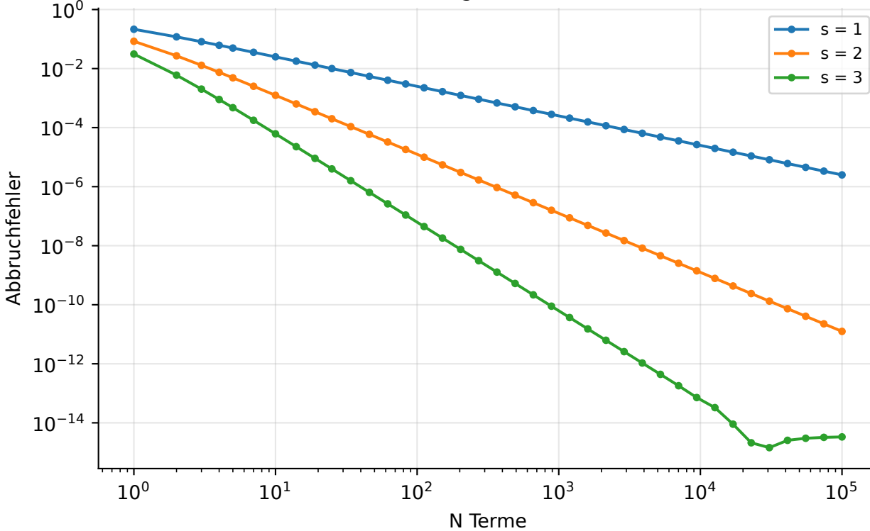
Reihenkonvergenz: Fehler \sim N^{-s}
