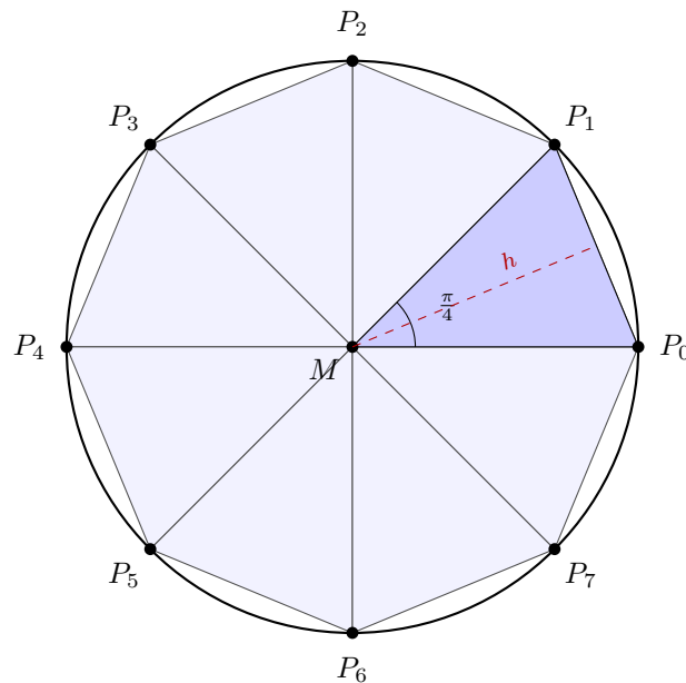
Abbildungung 11: Der Kreis nach drei Teilungen. Die acht Dreiecke T_k = \triangle MP_k P_{k+1} haben alle ihre Spitze in M (Winkel \frac{\pi}{4} ). Hervorgehoben ist T_0 mit der Höhe h = \cos \frac{\pi}{8} .
