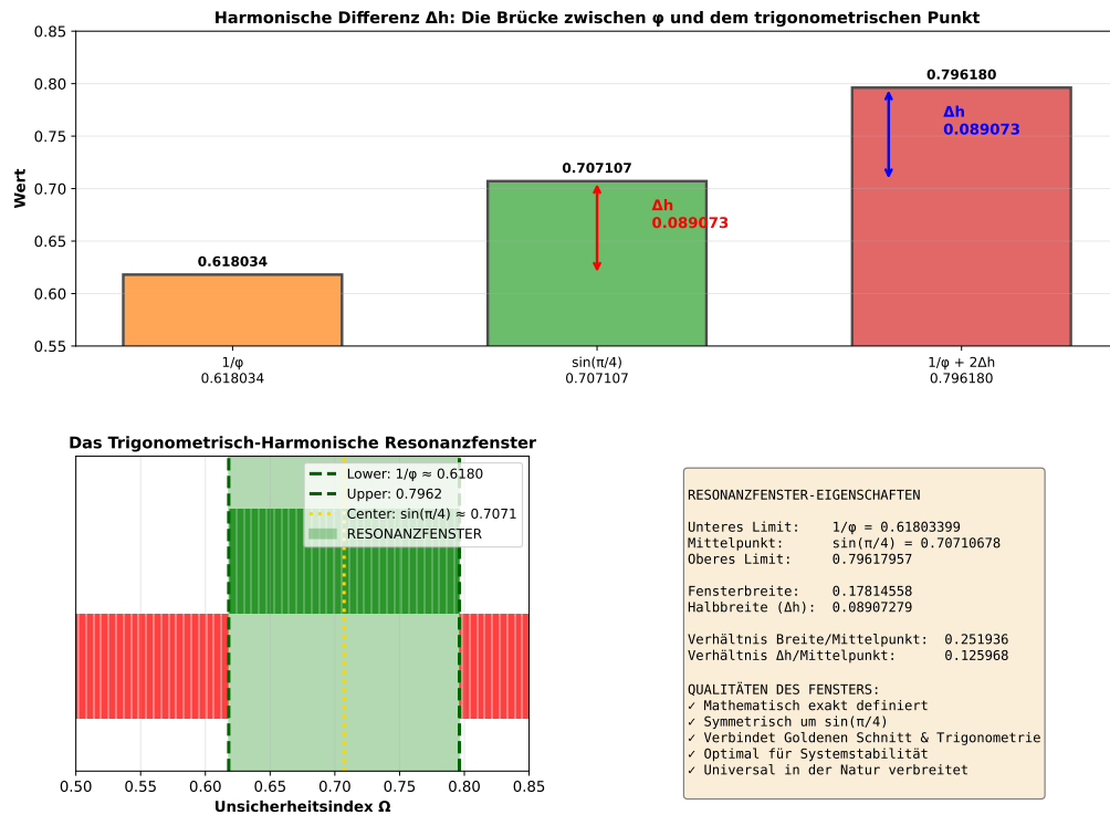
Abbildung 14: Der Plot zeigt, wie die Differenz zwischen 1/\phi und \sin(\pi/4) das dargestellte Resonanzfenster aufspannt.
