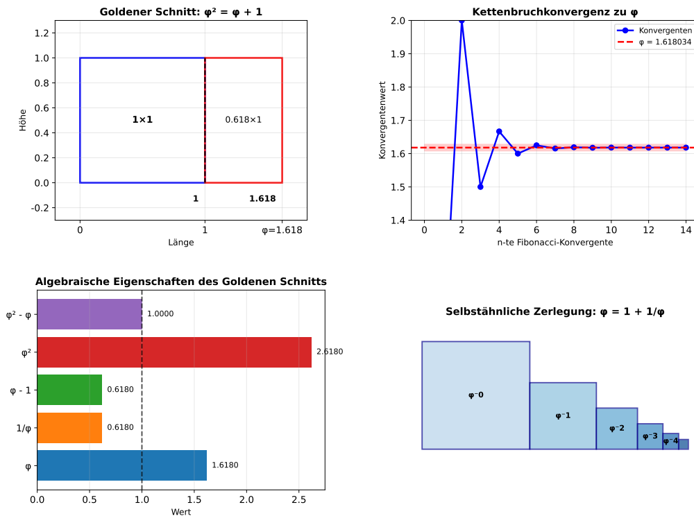
Abbildung 12: Der Plot zeigt die geometrische, algebraische und Fibonacci-basierte Struktur des Goldenen Schnitts.
