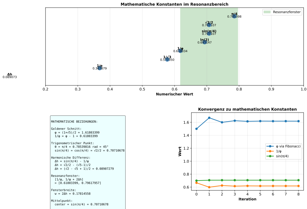
Abbildung 22: Der Plot vergleicht die zentralen mathematischen Konstanten und ihre Positionen im Resonanzbereich.
