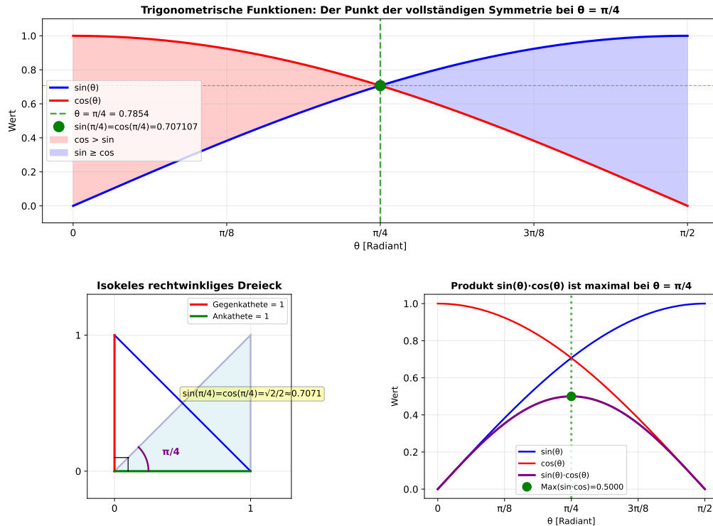
Abbildung 13: Der Plot macht den Gleichheitspunkt von Sinus und Kosinus bei \theta = \pi/4 geometrisch und analytisch sichtbar.
