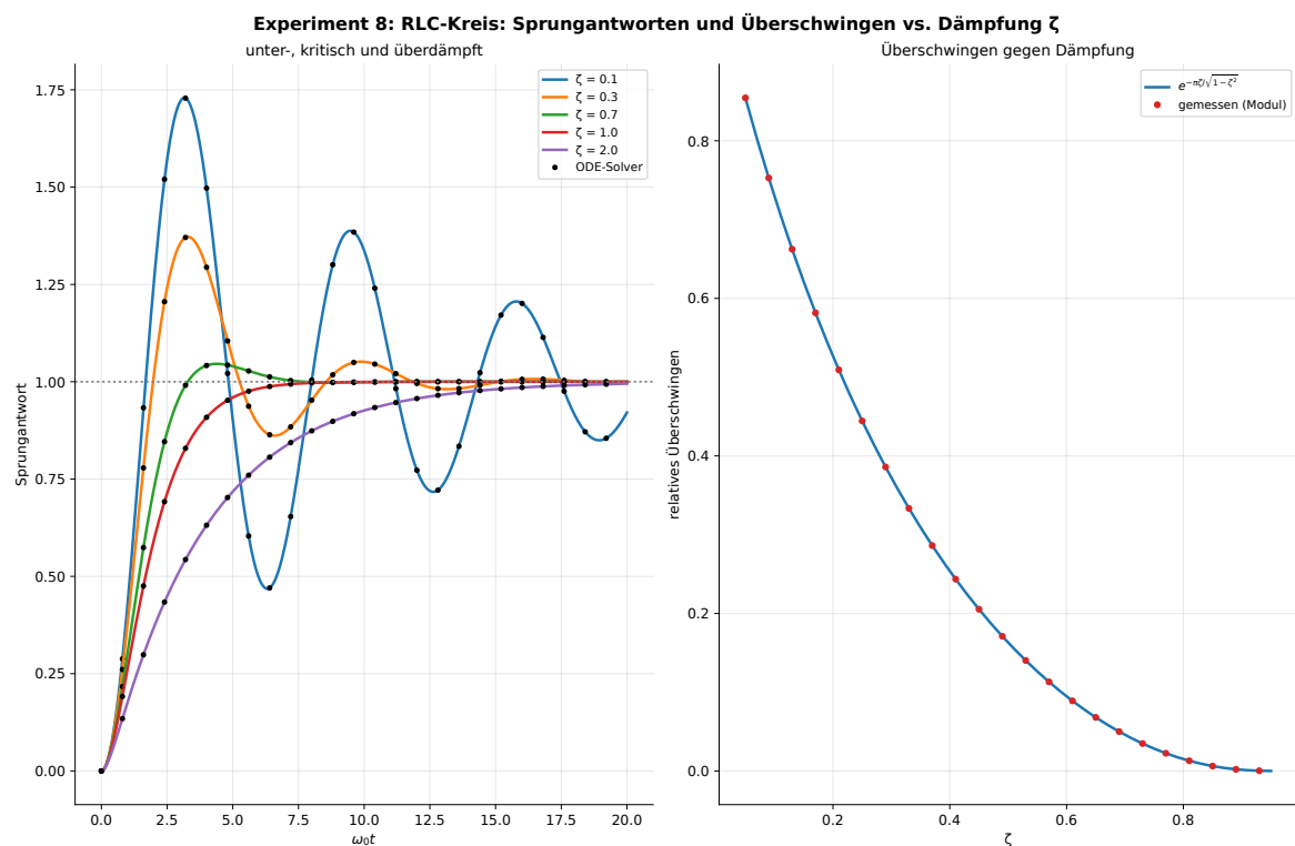
Abbildung 9: Die beiden Teilgrafiken vergleichen RLC-Sprungantworten und das relative Überschwngen als Funktion des Dämpfungsgrades.
