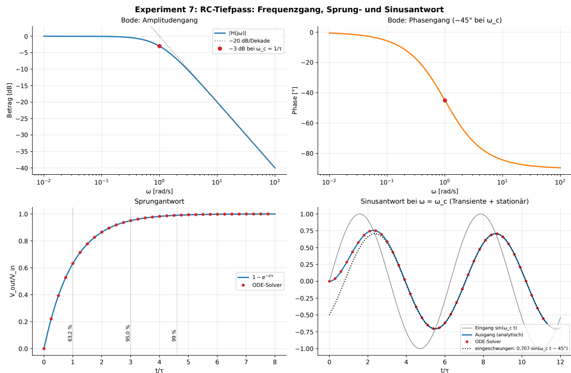
Abbildung 8: Die vier Teilgrafiken zeigen Betrag und Phase des Frequenzgangs sowie Sprung- und Sinusantwort des RC-Tiefpasses.
