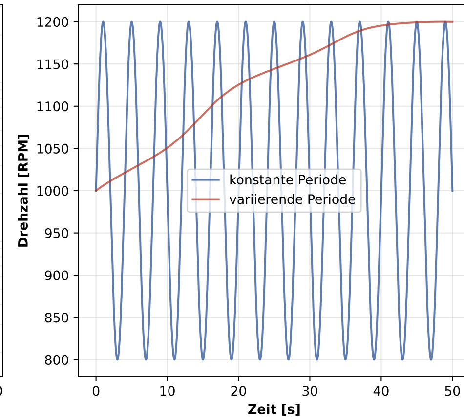
Drehzahl-Vergleich
