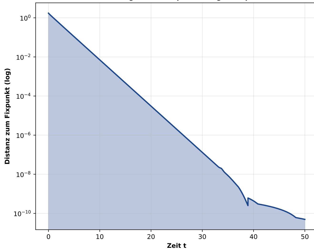
Konvergenz zur Fixpunktmenge \text{Fix}(\varphi)
