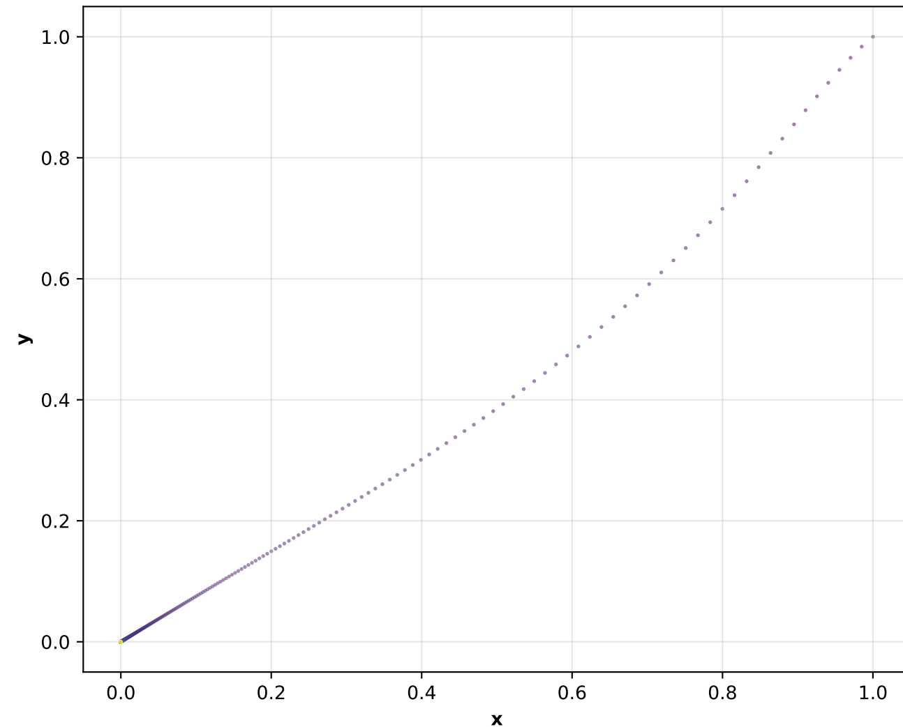
Bifurkation der Fixpunkte
