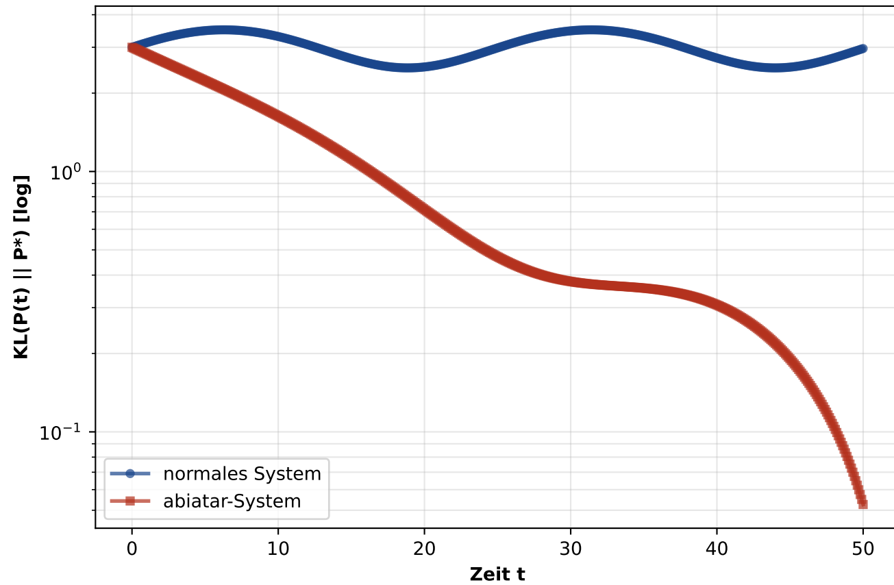
KL-Divergenz zur Fixpunktverteilung
